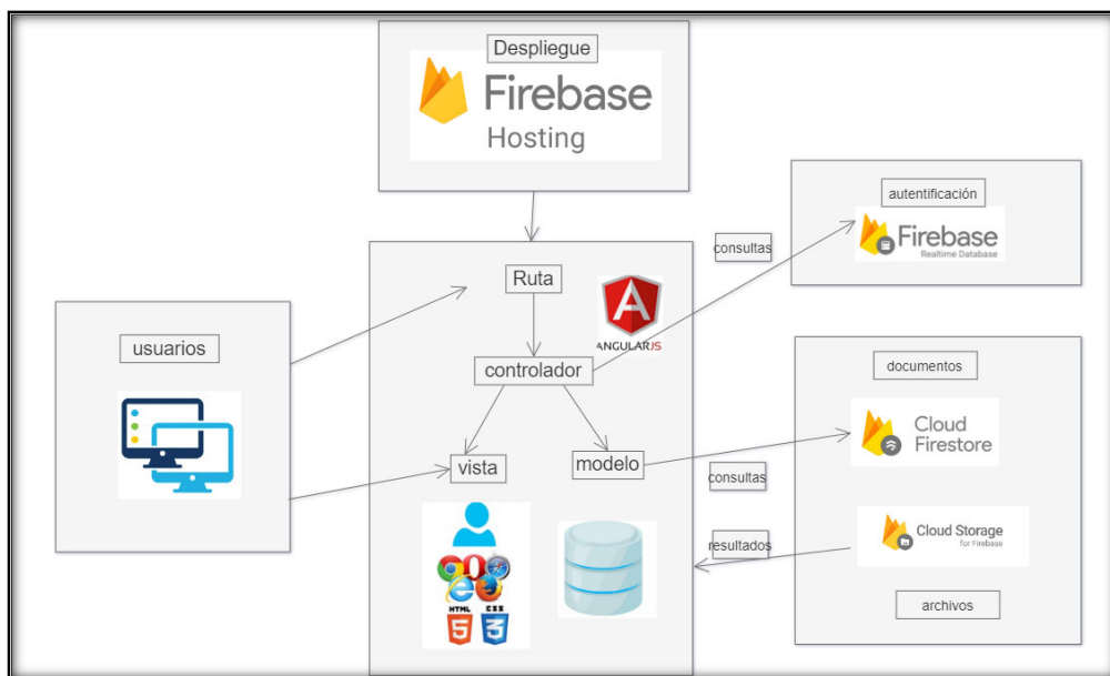
Fig. 2: Patrón arquitectónico.
