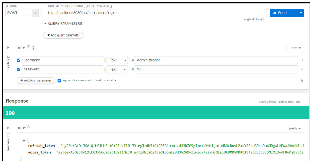
Fig. 79: Método POST inicio de sesión en Talend API Tester .
