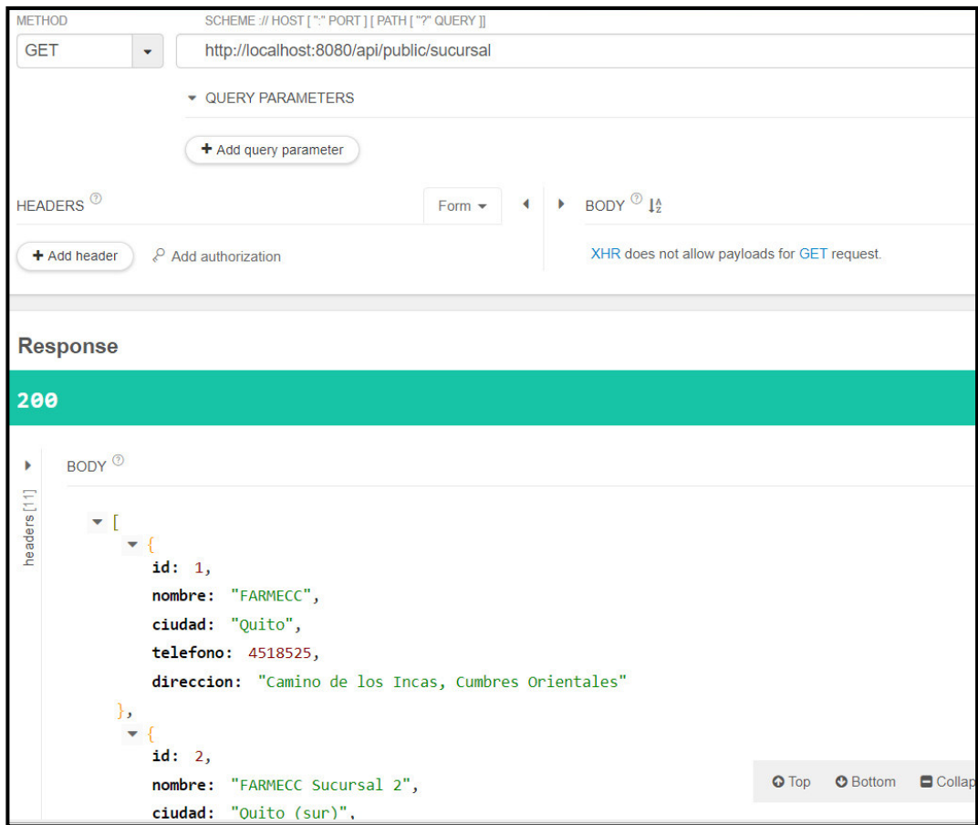
Fig. 78: Método GET sucursales en Talend API Tester .
