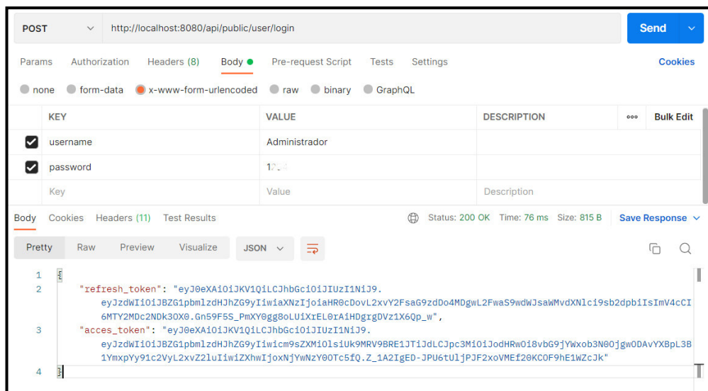
Fig. 19: Método POST para inicio de sesión.
