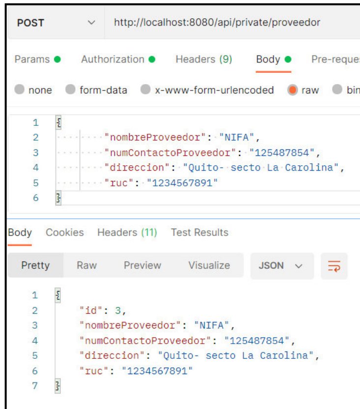
Fig. 27: Método POST para agregar proveedores.
