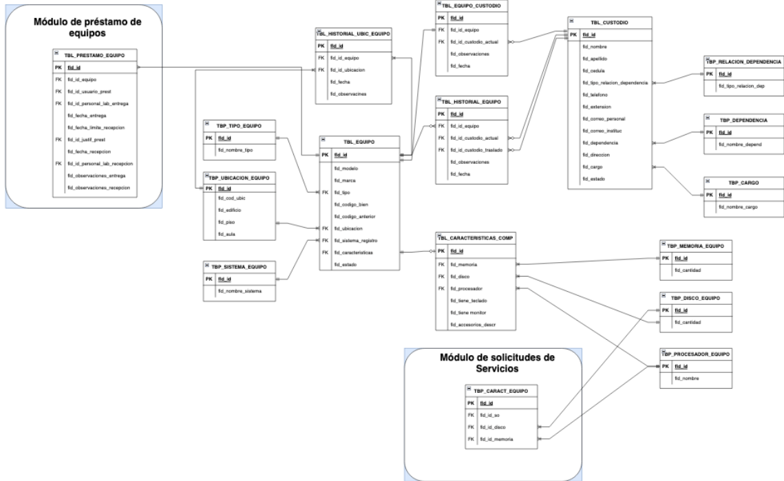
Diagrama entidad relación de la base de datos del módulo de inventario
