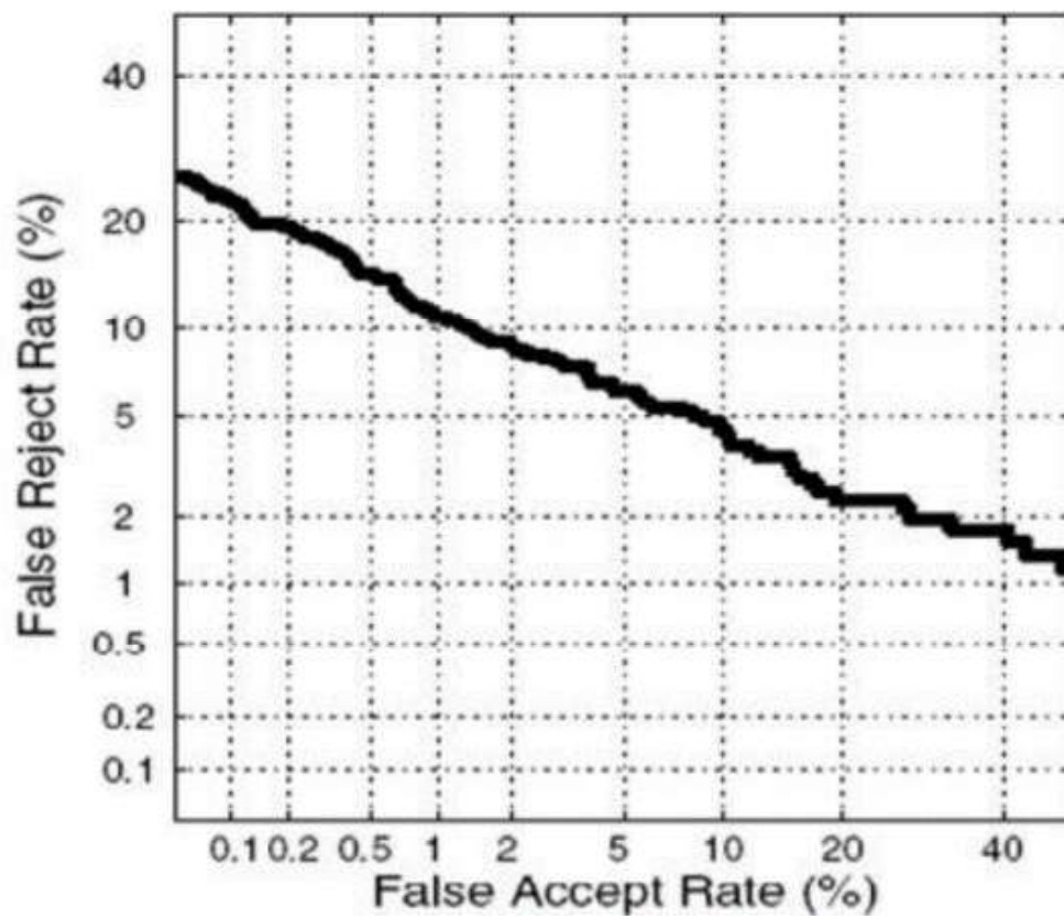
Figura 1.16. Rendimiento de un sistema biométrico resumido en un gráfico DET [19].
