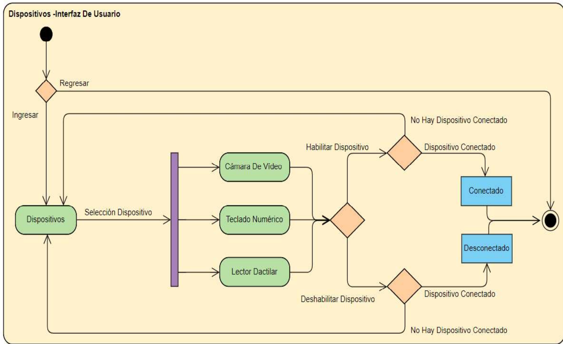
Figura 2.21. Diagrama de actividades de la administración de dispositivos.
