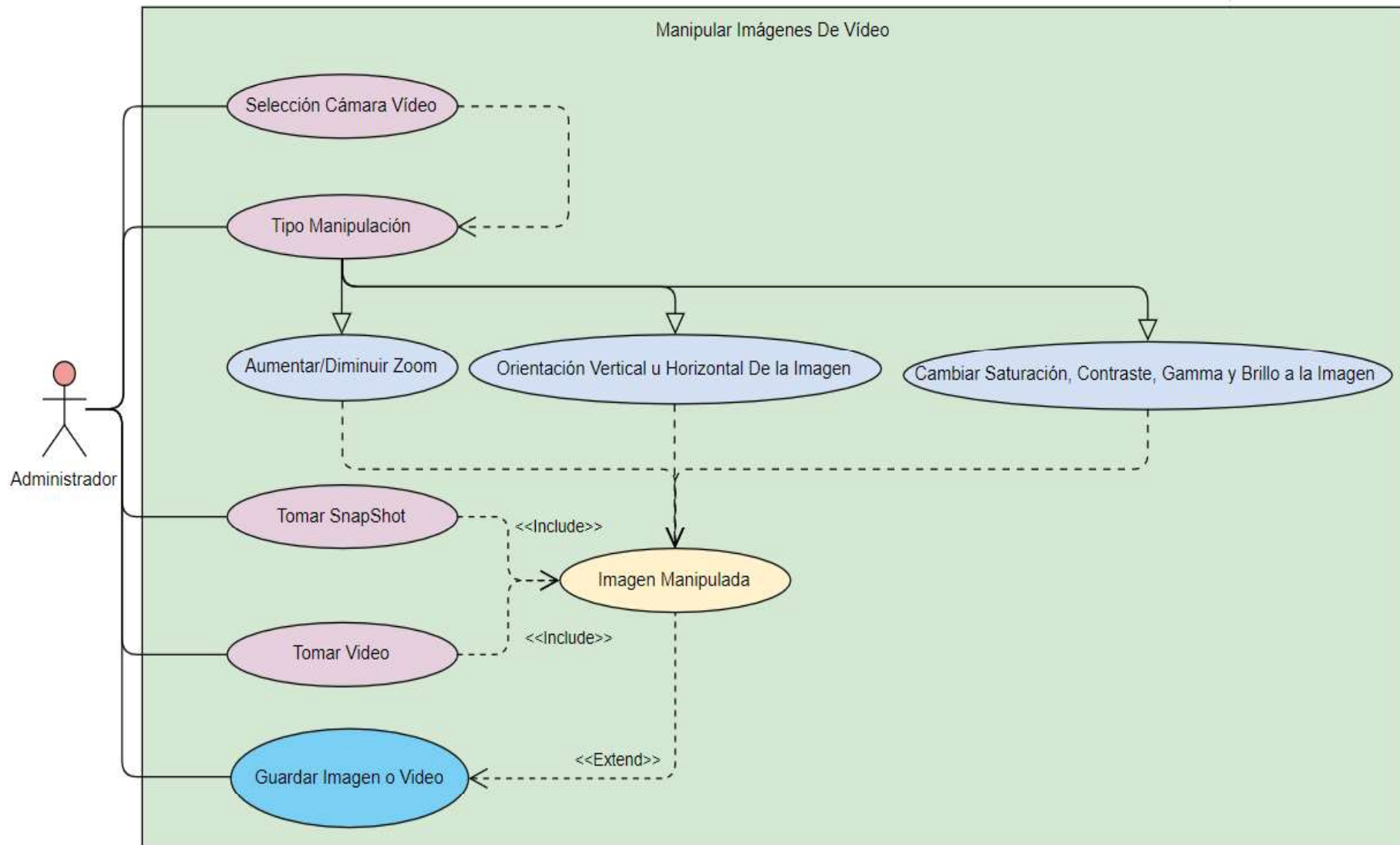
Figura 2.11. Diagrama de caso de uso para la manipulación de las imágenes de video.
