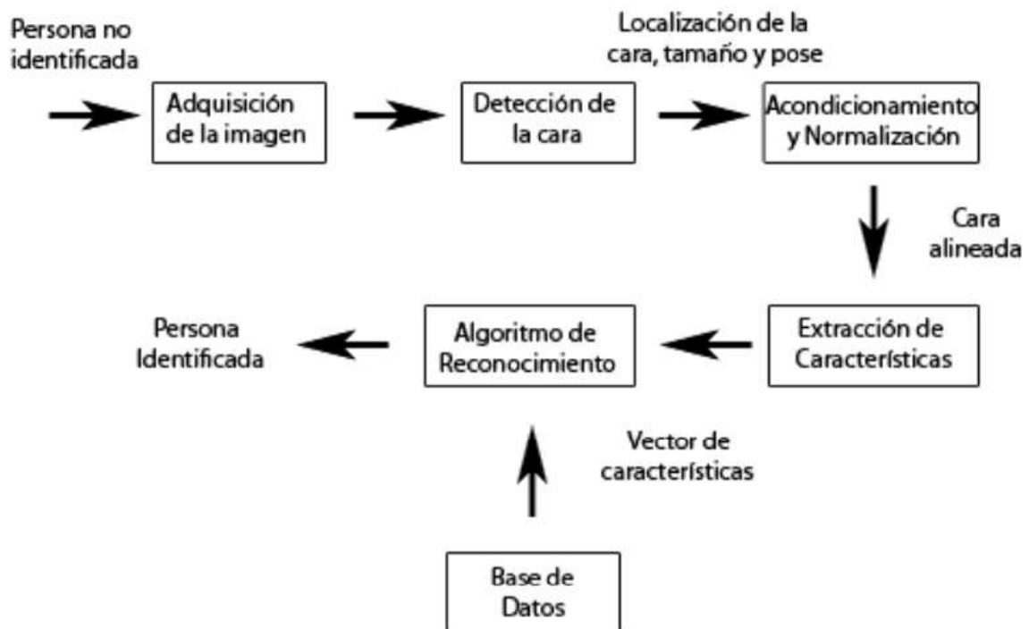
Figura 1.21. Procedimiento para el reconocimiento facial [23].
