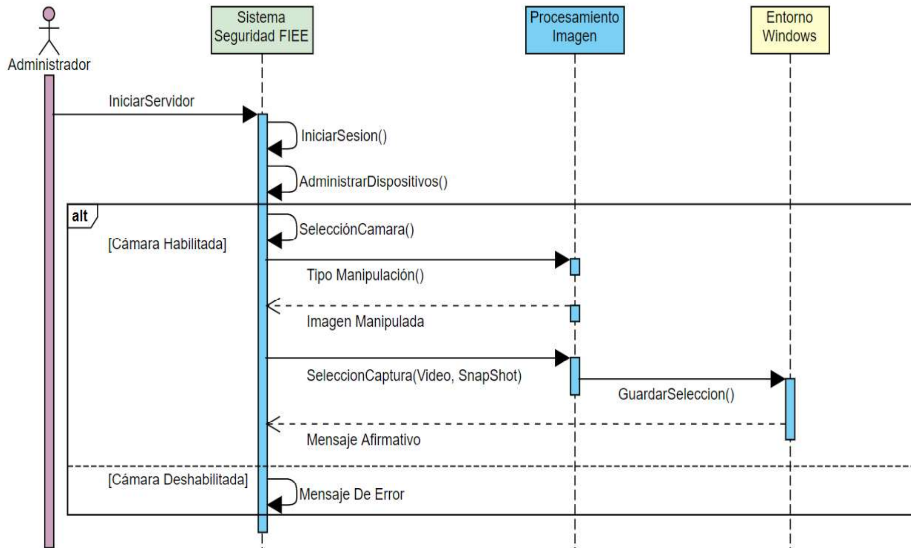
Figura 2.12. Diagrama de secuencia para la manipulación de las imágenes de video.
