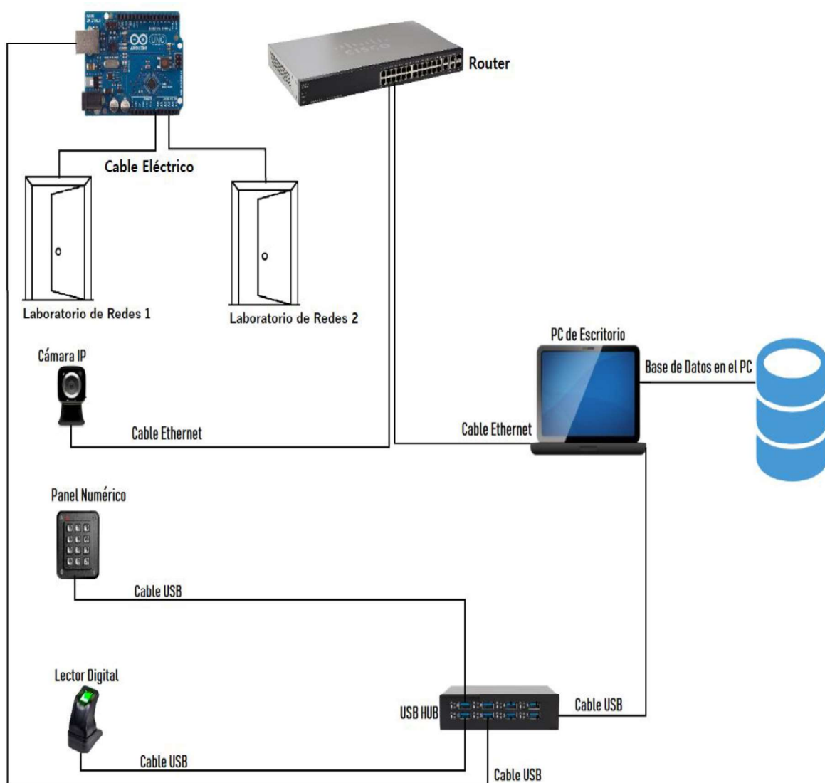
Figura 2.58. Implementación del sistema de seguridad.
