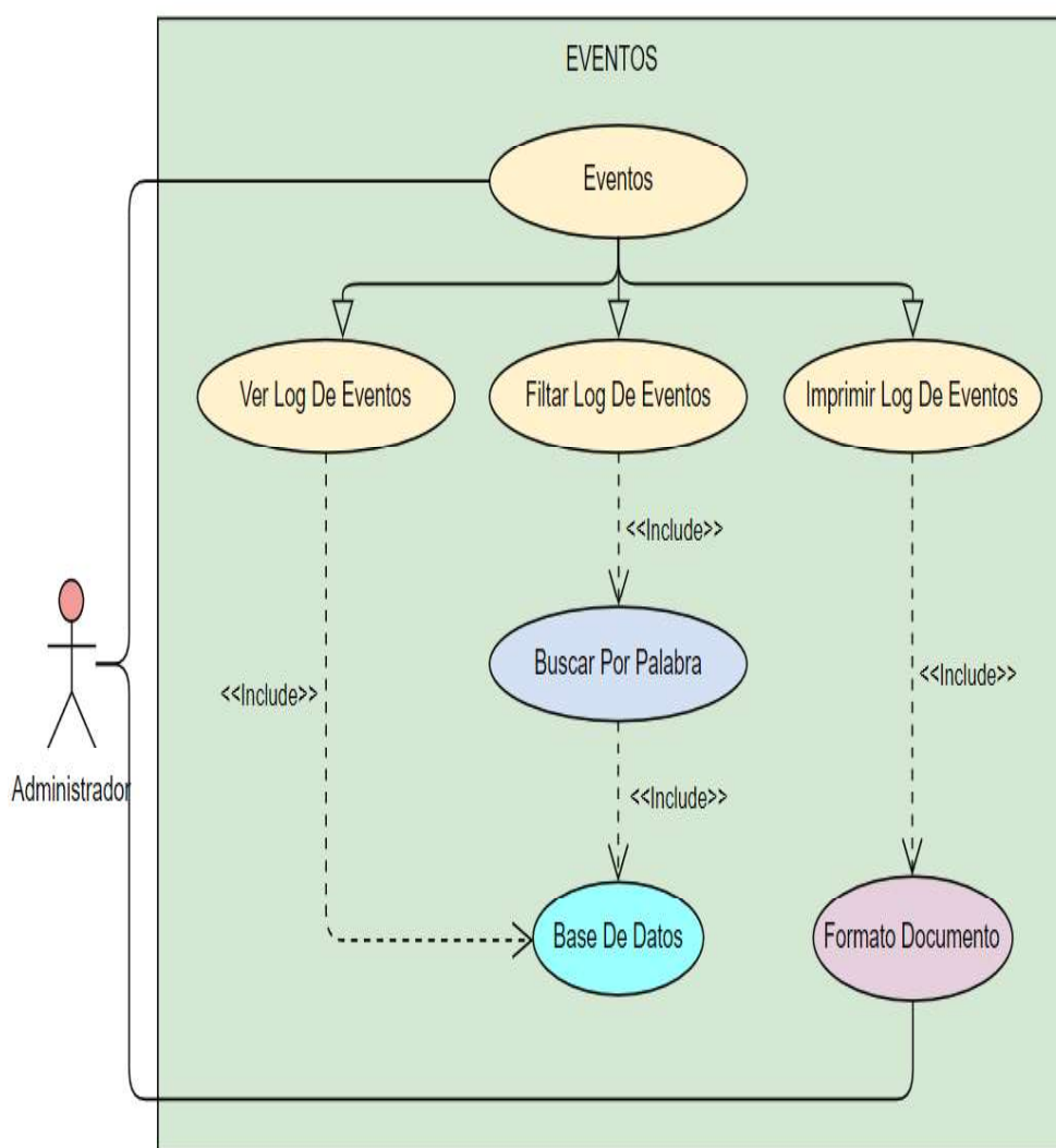
Figura 2.7. Diagrama de caso de uso administración del log de eventos.
