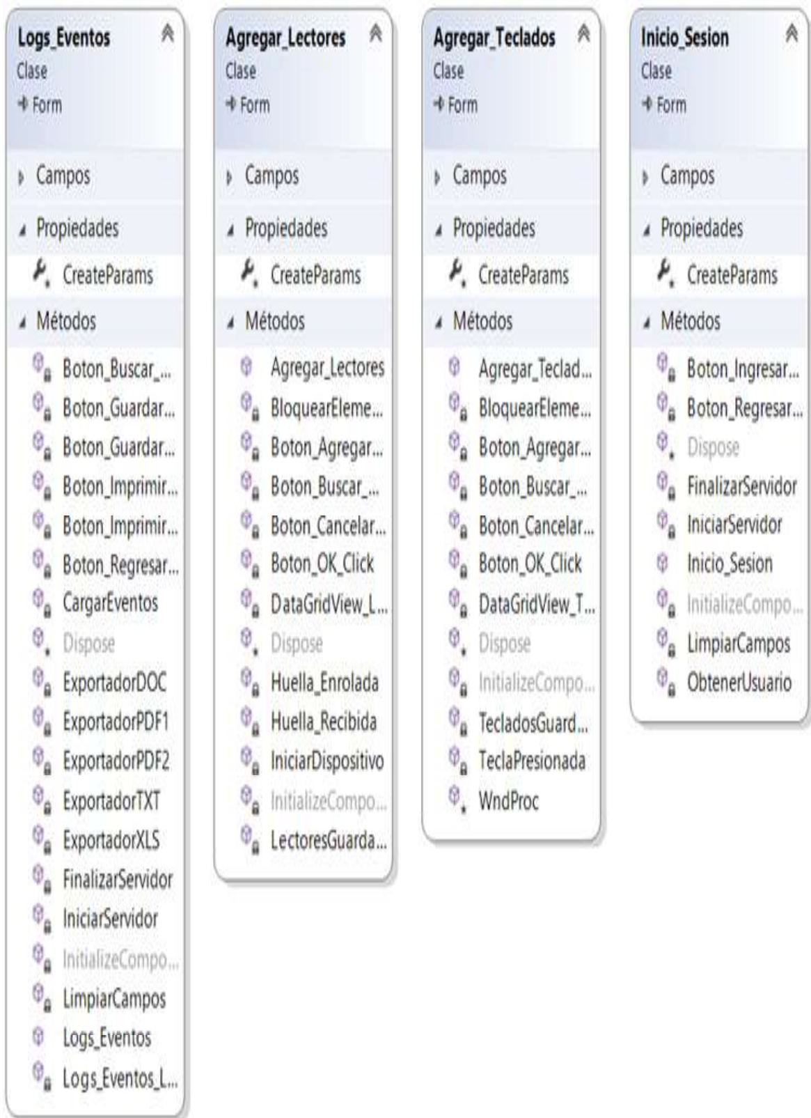
Figura 2.14. Diagrama de clases de la interfaz de usuario.
