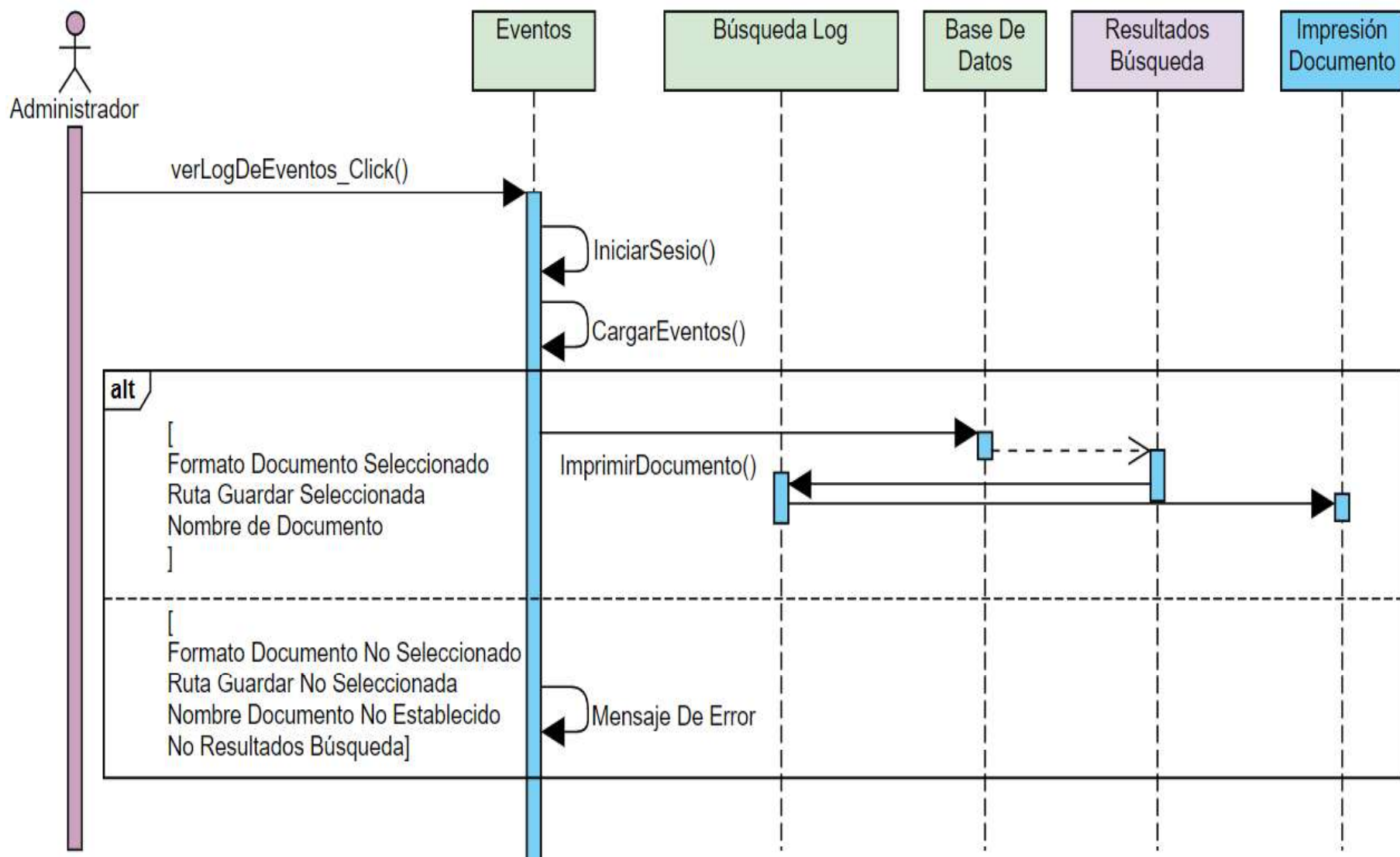
Figura 2.8. Diagrama de secuencia del log de eventos.
