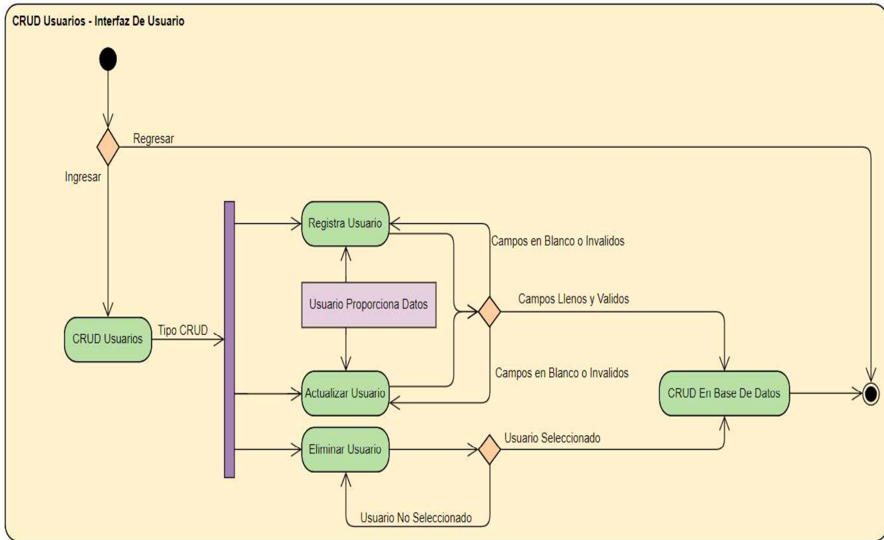
Figura 2.19. Diagrama de actividades del CRUD usuarios.
