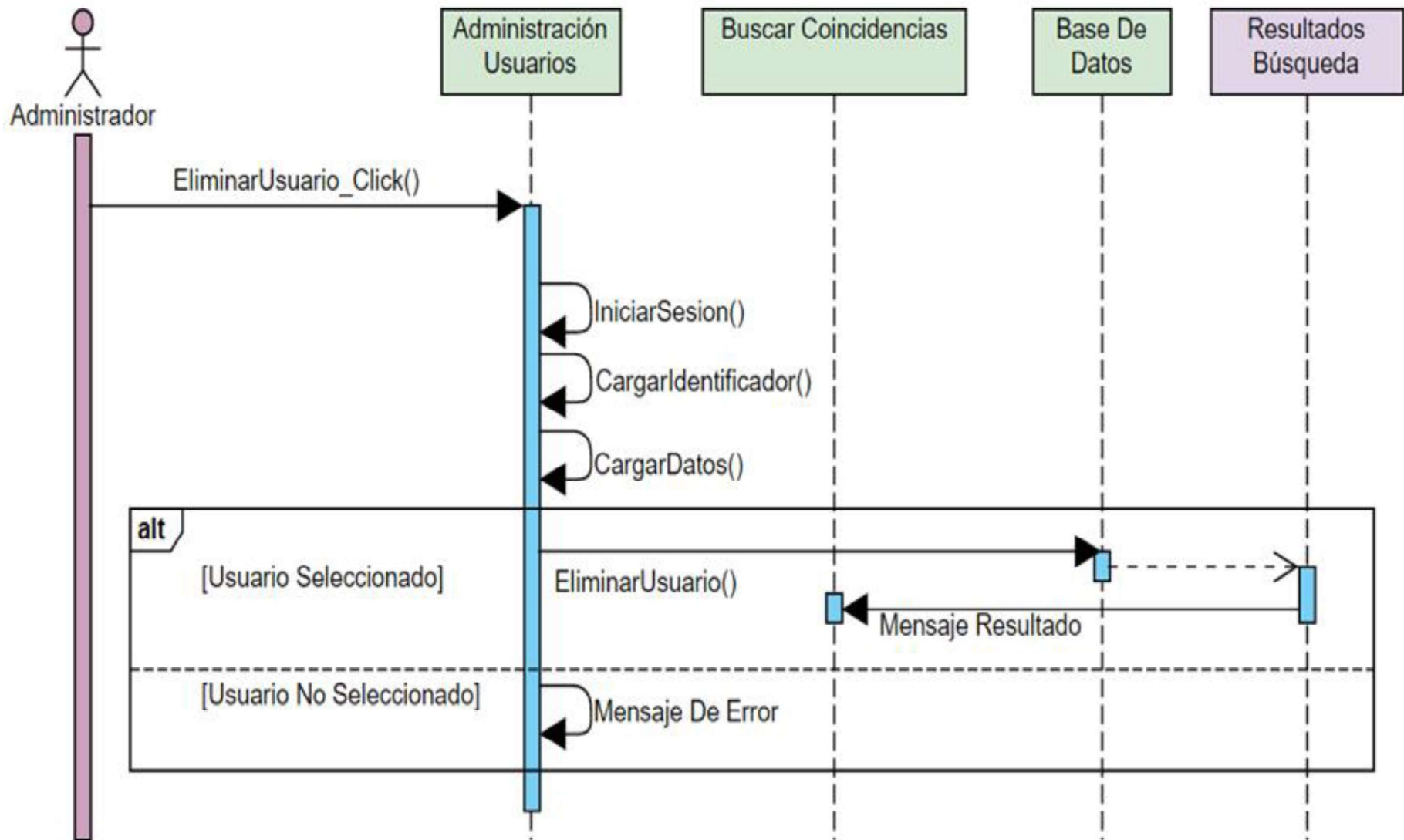
Figura 2.6. Diagrama de secuencia de la eliminación de usuarios.
