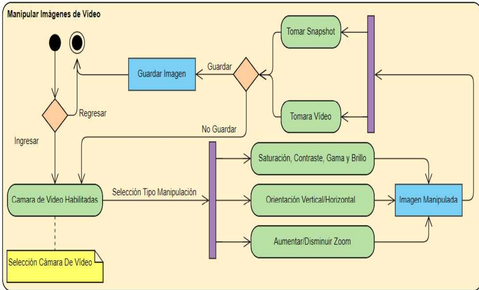
Figura 2.22. Diagrama de actividades de la manipulación de las imágenes de Video.
