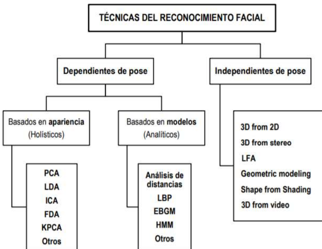
Figura 1.24. Técnicas del reconocimiento facial [8].
