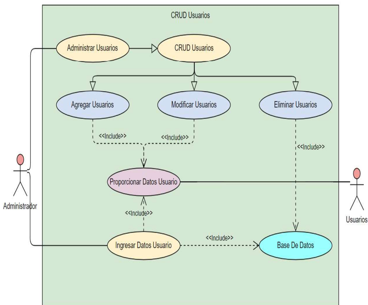
Figura 2.4. Diagrama de caso de uso del CRUD de usuarios.
