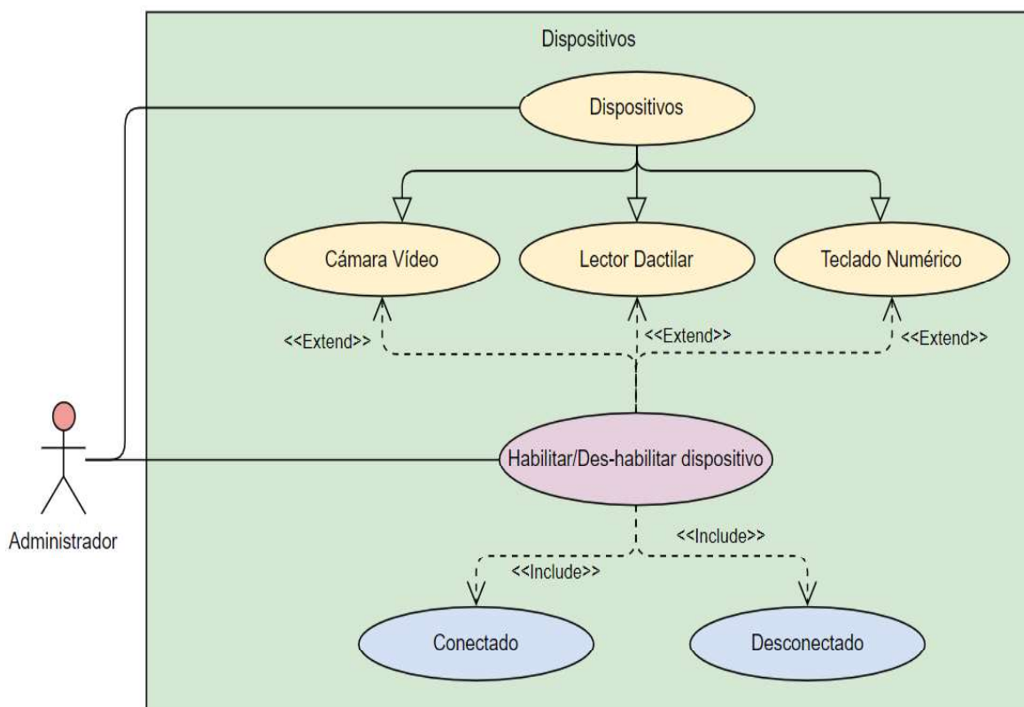
Figura 2.9. Diagrama de caso de uso para la administración de dispositivos.
