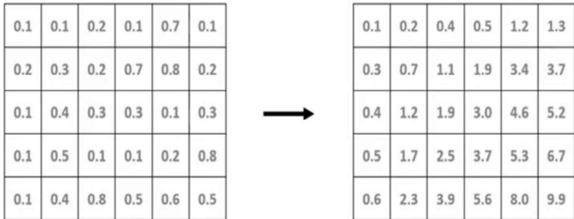
Figura 1.18. Cambio de imagen original a una imagen integral.
