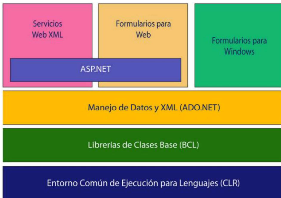
Figura 1.7. Biblioteca de clases base [32].
