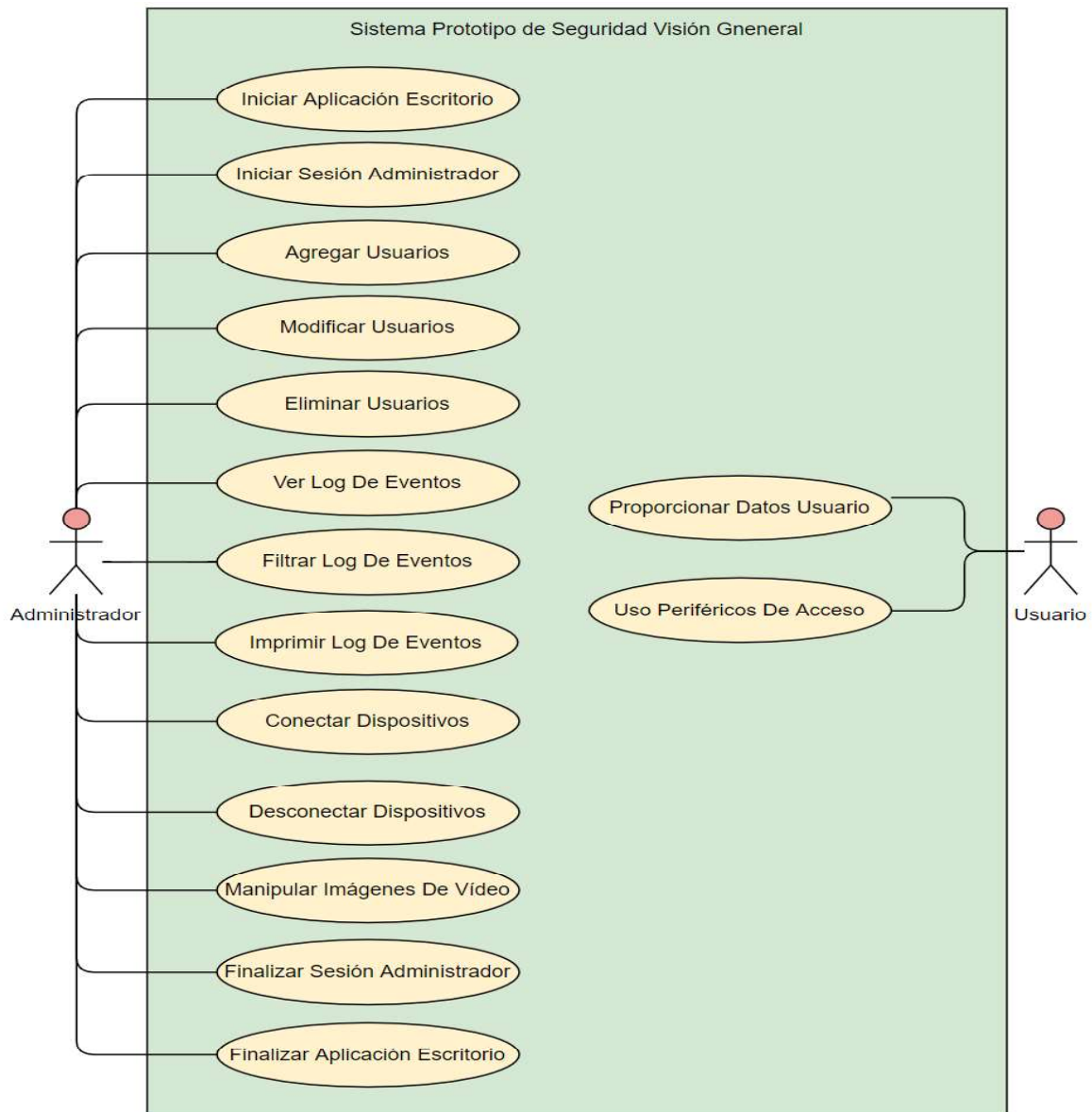
Figura 2.1. Diagrama de caso de uso general.
