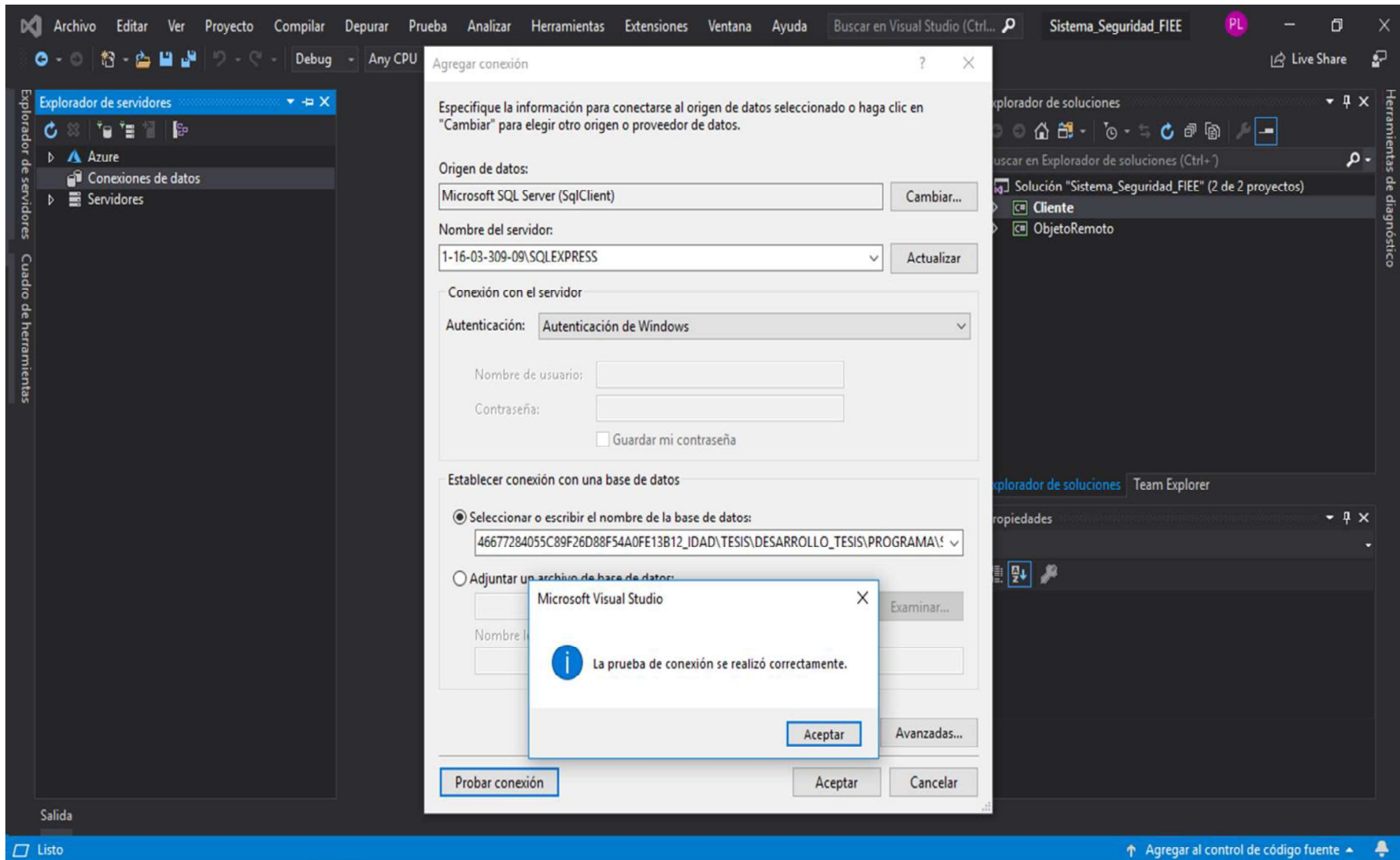
Figura 3.10. Conexión de la base de datos en el nuevo computador.
