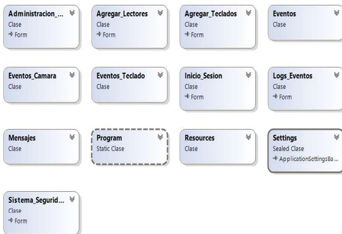
Figura 2.13. Diagrama de clases de la interfaz de usuario y la lógica de negocios.
