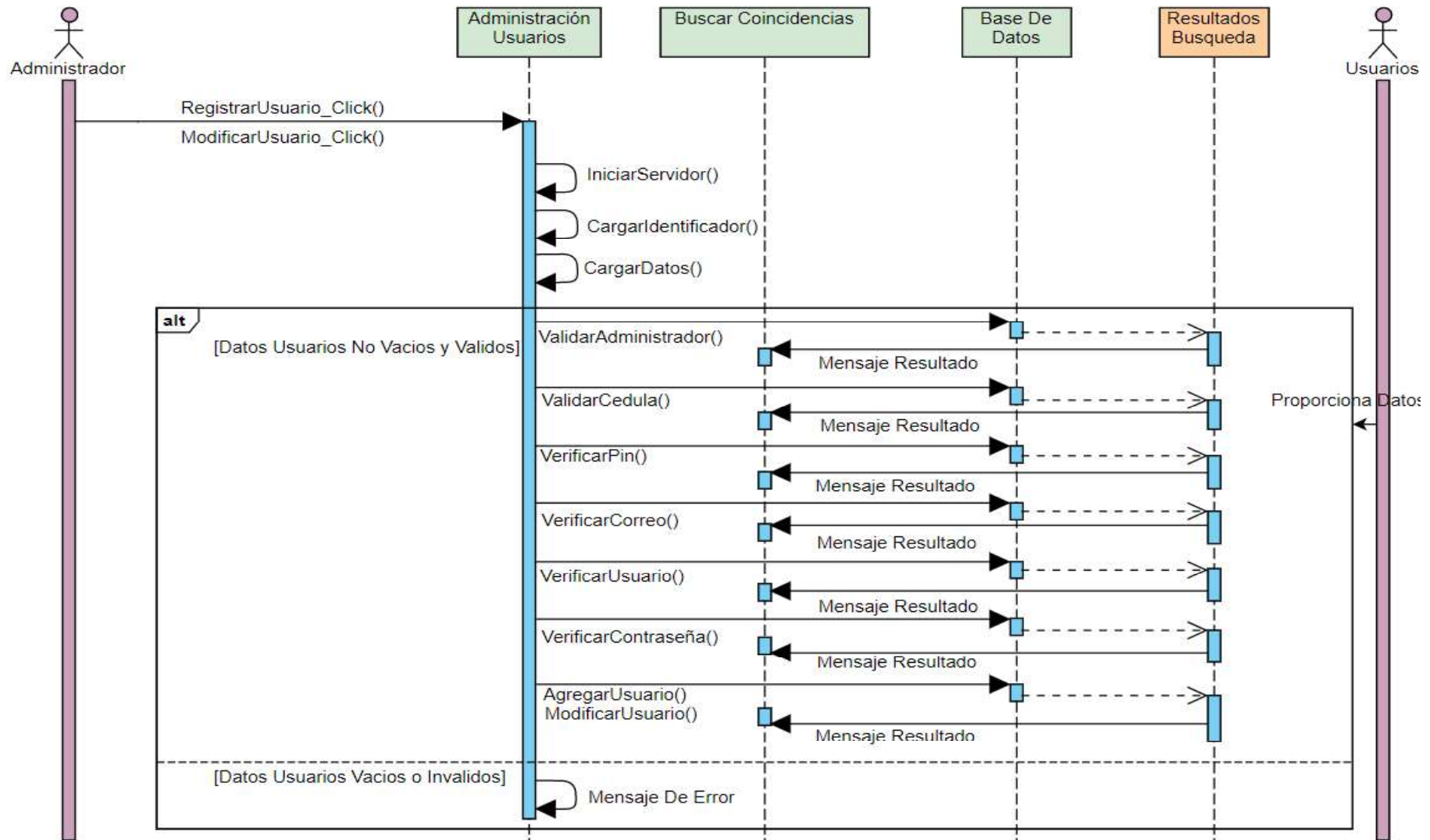
Figura 2.5. Diagrama de secuencia del registro y modificación de usuarios.
