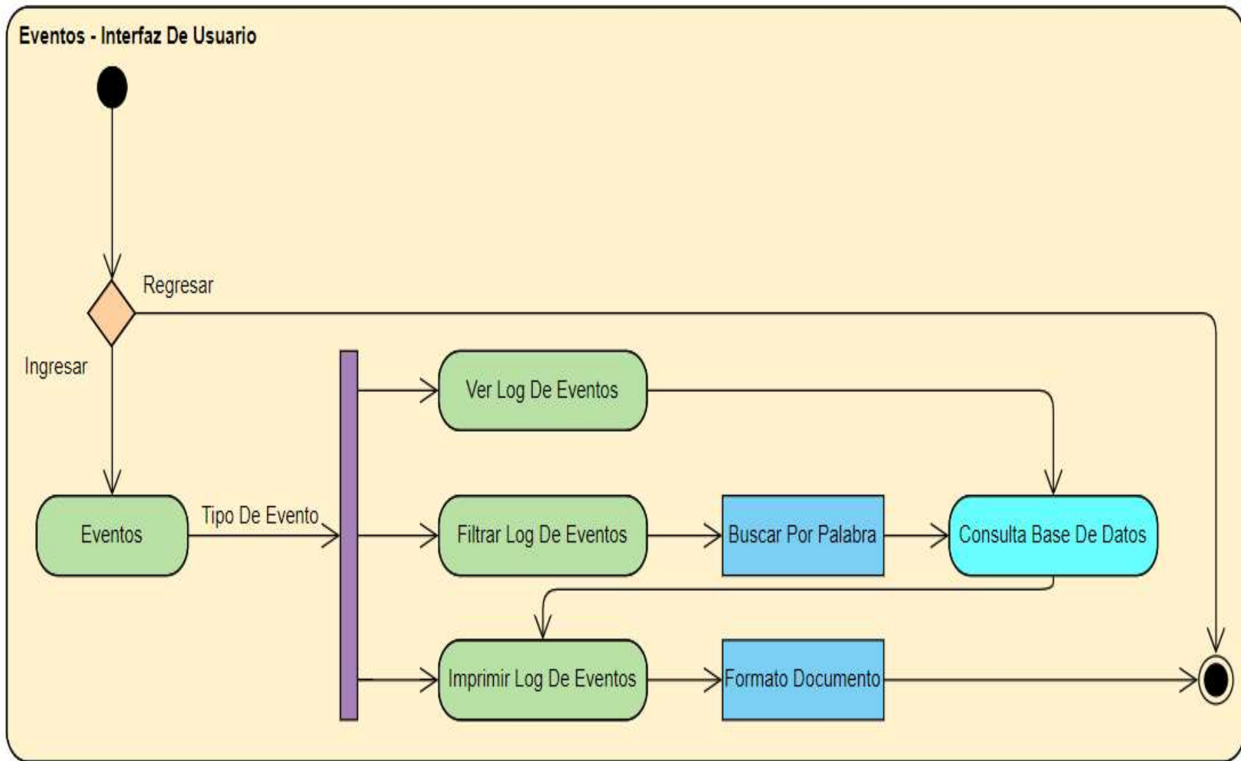
Figura 2.20. Diagrama de actividades del log de eventos.
