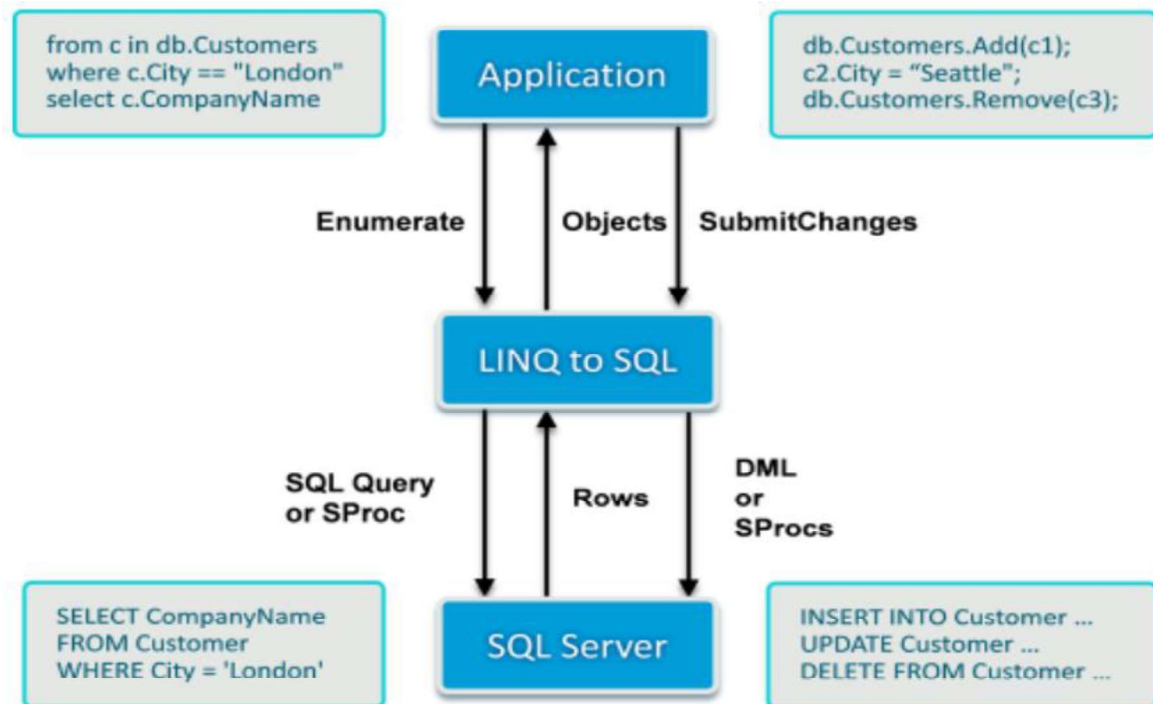
Figura 1.10. Mapeador de objetos relacionales [39].
