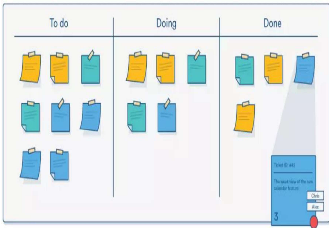
Figura 1.34. Tablero Kanban [50].
