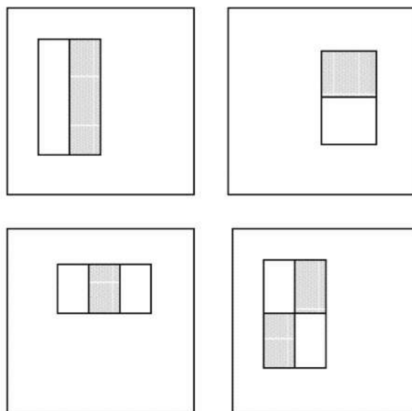
Figura 1.19. Características haar [17].
