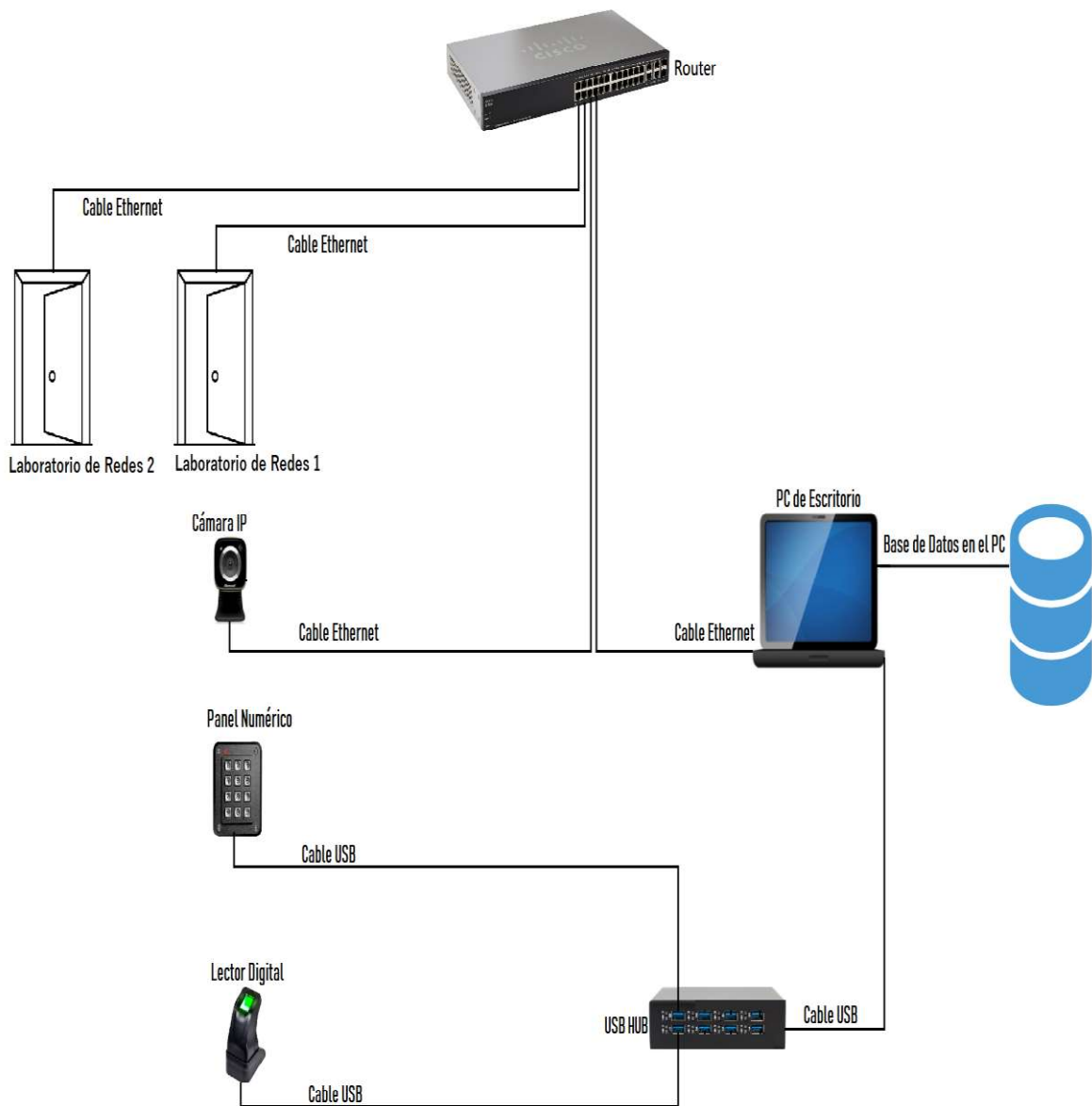
Figura 1.1. Prototipo del sistema de seguridad basado en reconocimiento facial.
