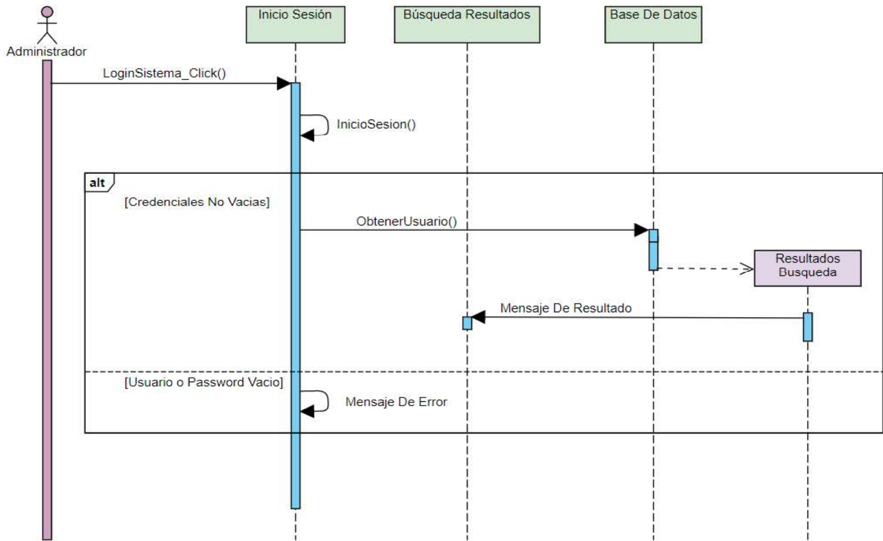
Figura 2.3. Diagrama de secuencia del inicio de sesión.
