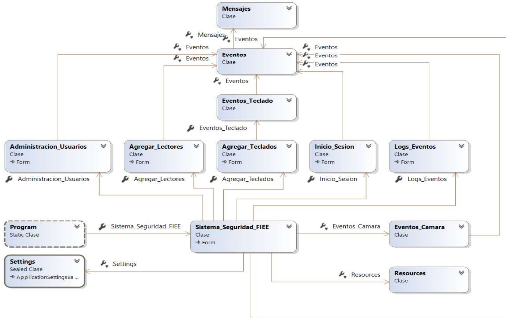
Figura 2.15. Diagrama de clases lógica de negocios.
