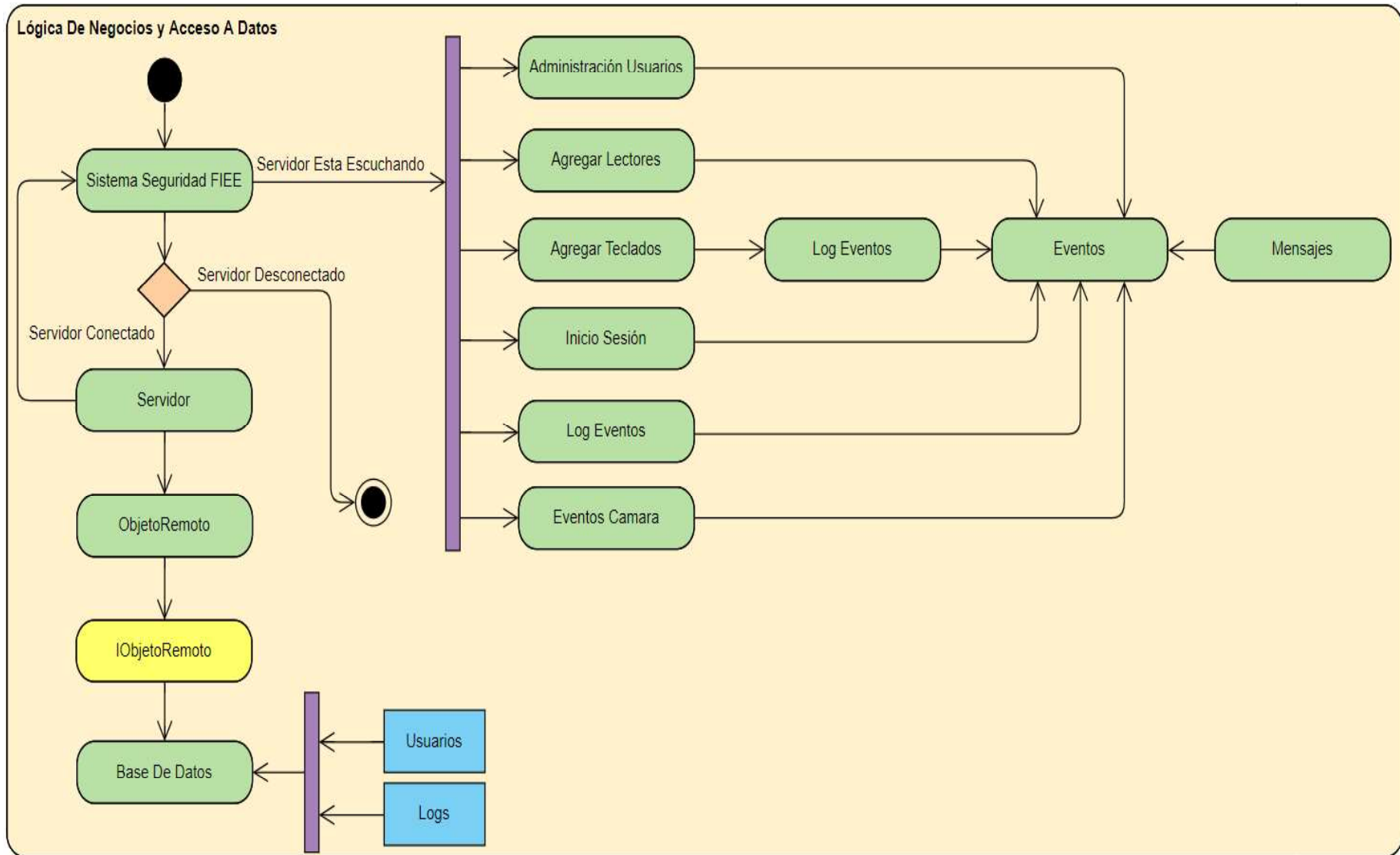
Figura 2.23. Diagrama de actividades lógica de negocios y acceso a datos.
