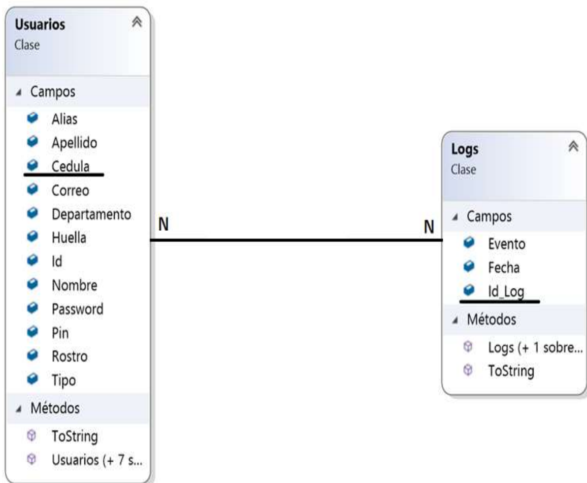
Figura 2.24. Diagrama entidad relación del módulo base de datos.
