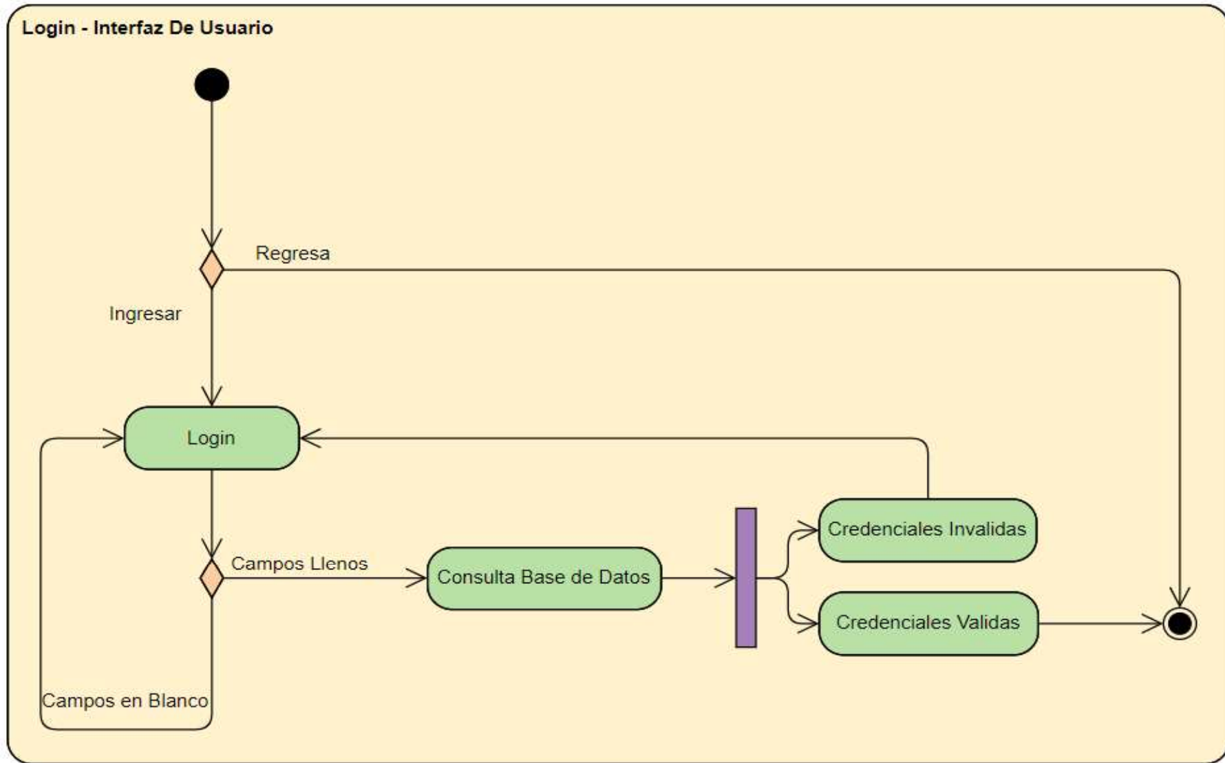
Figura 2.18. Diagrama de actividades del login.
