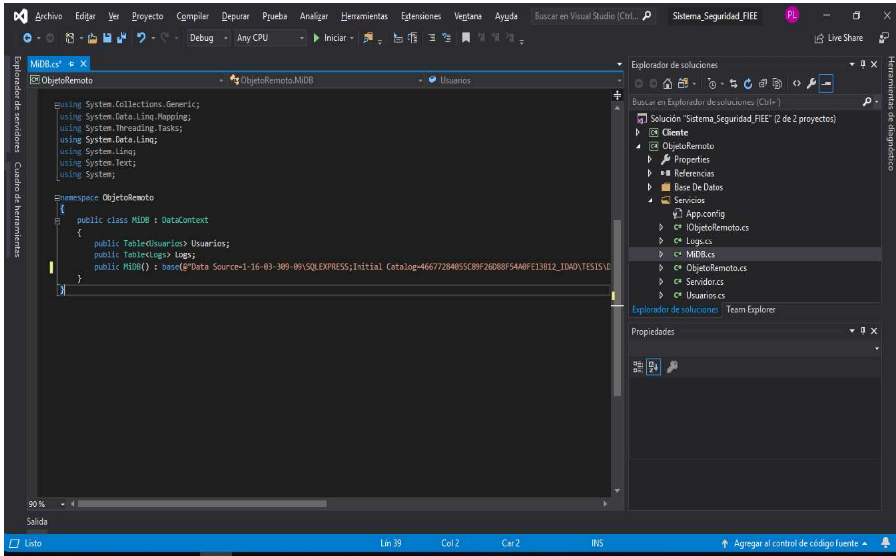
Figura 3.11. Actualizando la cadena de conexión de la base de datos.
