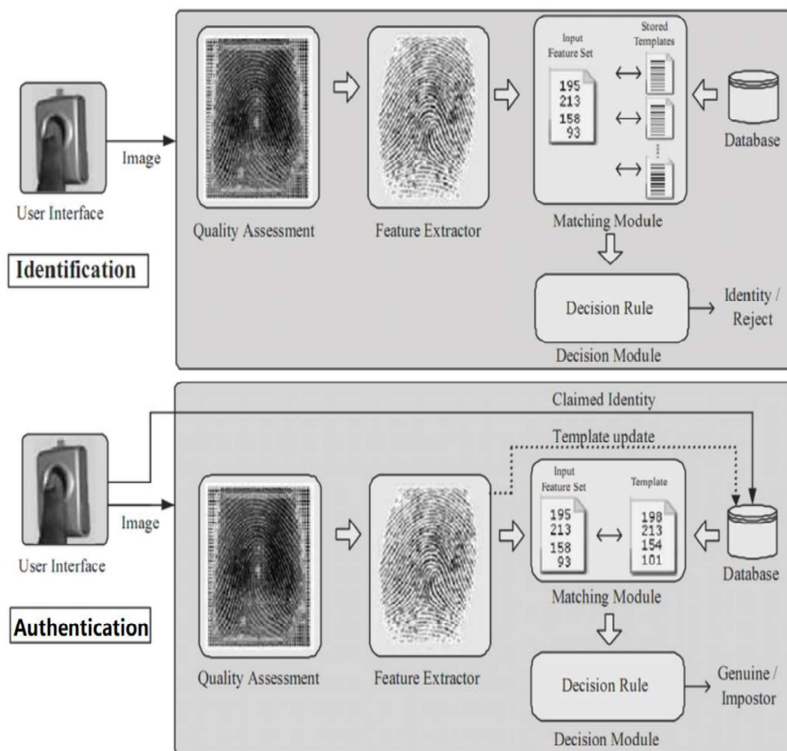
Figura 1.15. Identificación (arriba) y autenticación (abajo), diferencias entre las fases [19].
