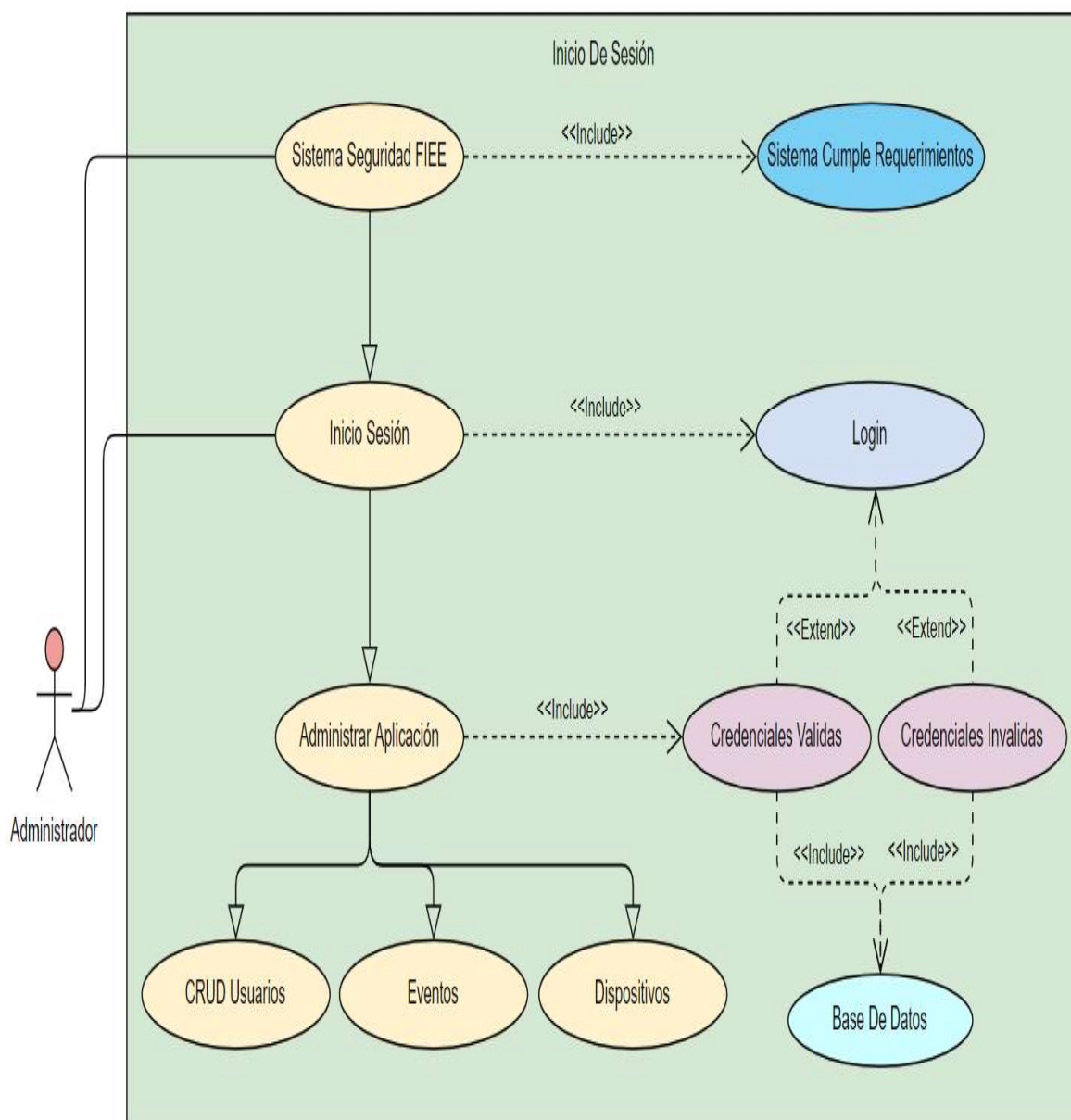
Figura 2.2. Diagrama de caso de uso del inicio de sesión.
