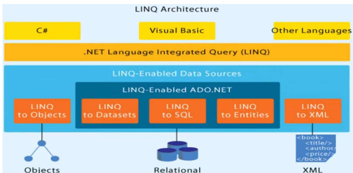
Figura 1.11. Arquitectura LINQ [3].
