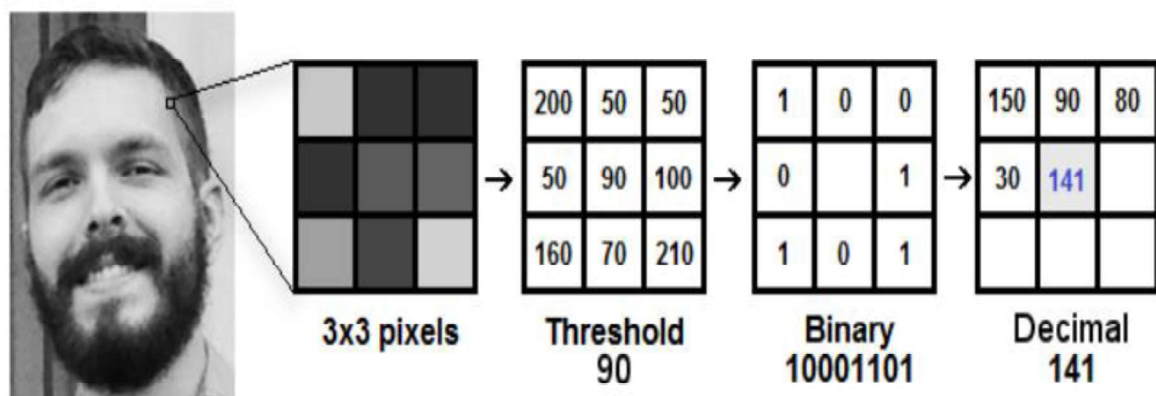
Figura 1.28. Operación LBP aplicada a una imagen [49].
