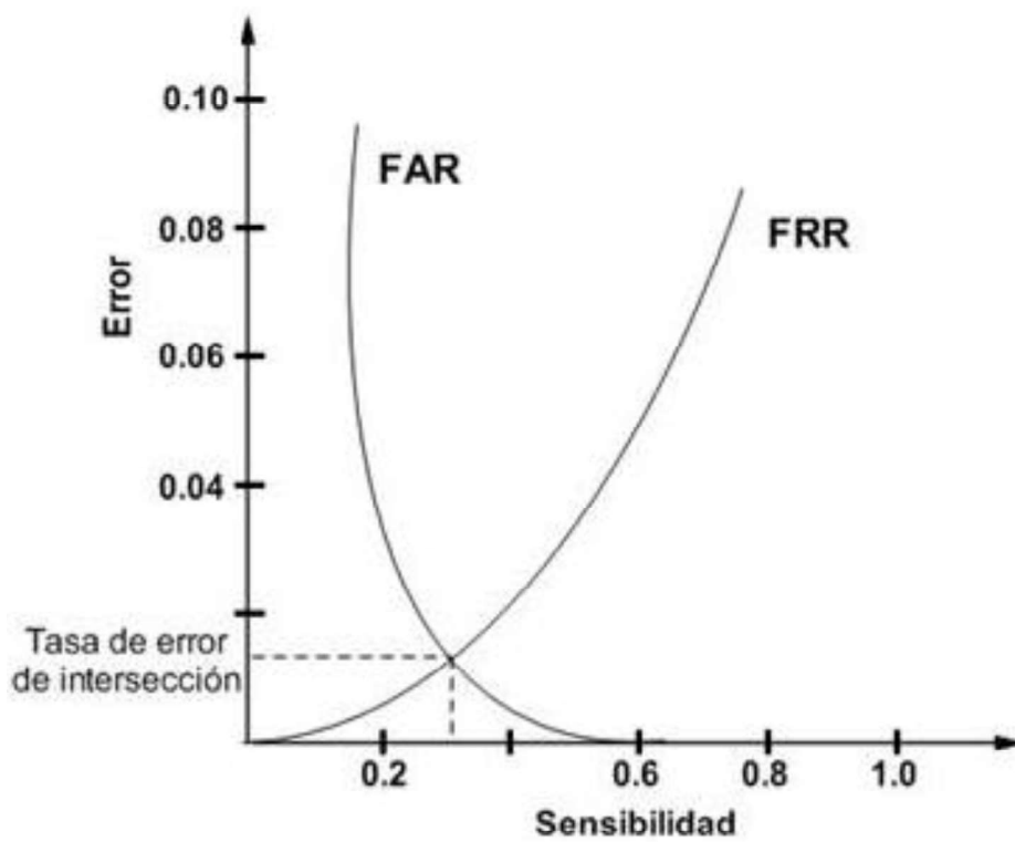
Figura 1.17. Sensibilidad del sistema biométrico.
