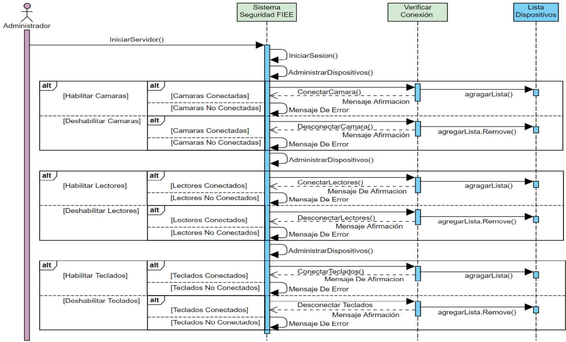
Figura 2.10. Diagrama de secuencia para la administración de dispositivos.
