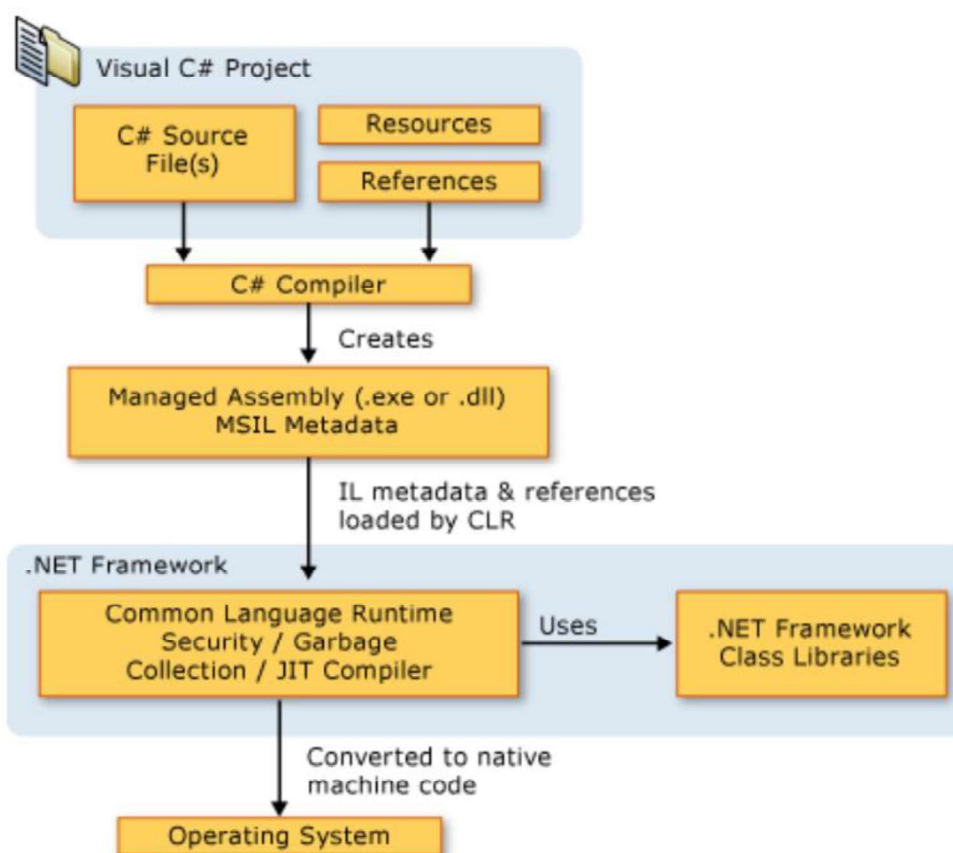
Figura 1.9. Compilación y creación del archivo ejecutable en C# [37].
