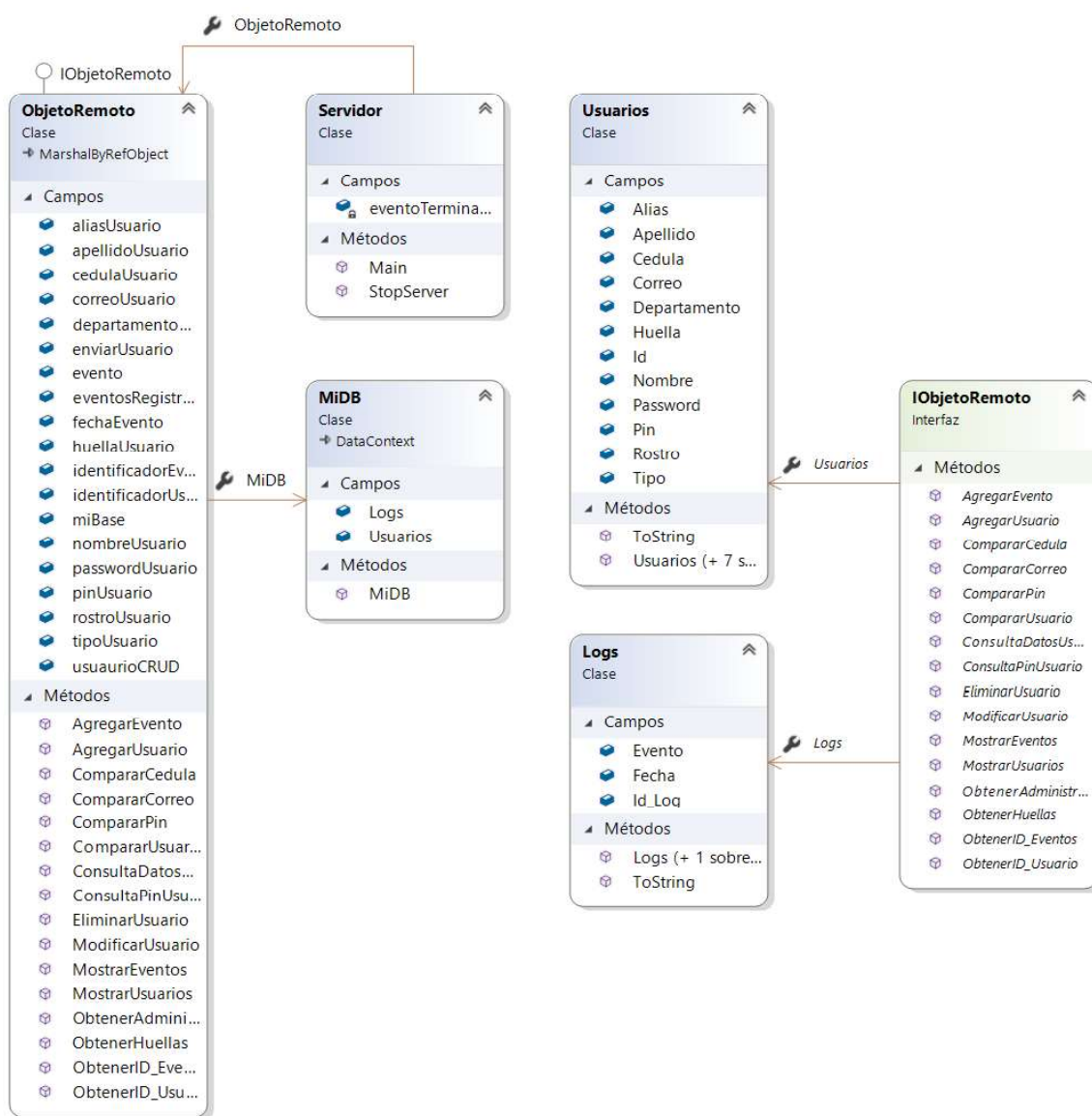
Figura 2.16. Diagrama de clases del acceso a datos y servidor.
