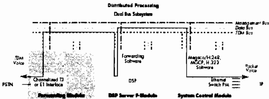
Figura 3.17 Arquitectura de bus redundante de la Pasarela de Encaminamiento Alcatel 7505 [10].
