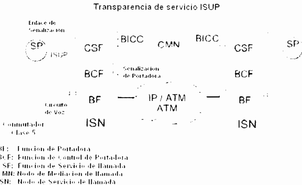
Figura 2.19 Arquitectura de la Red BICC CS1 [18].
