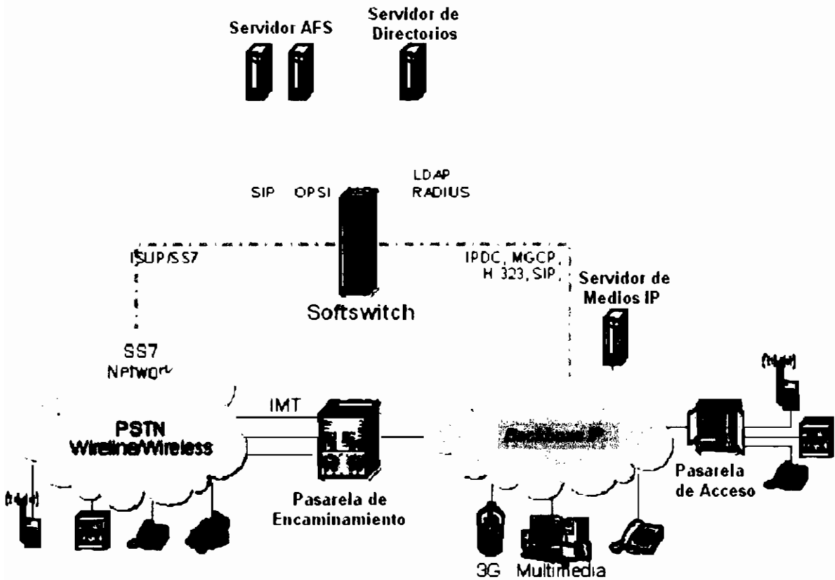
Figura 3.5 Diagrama de Red NGN con Inteligencia Centralizada [39].
