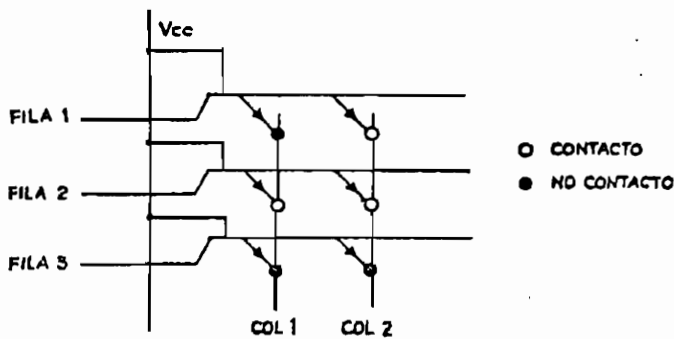
Figura 1.2 Matriz de diodos. [9]
