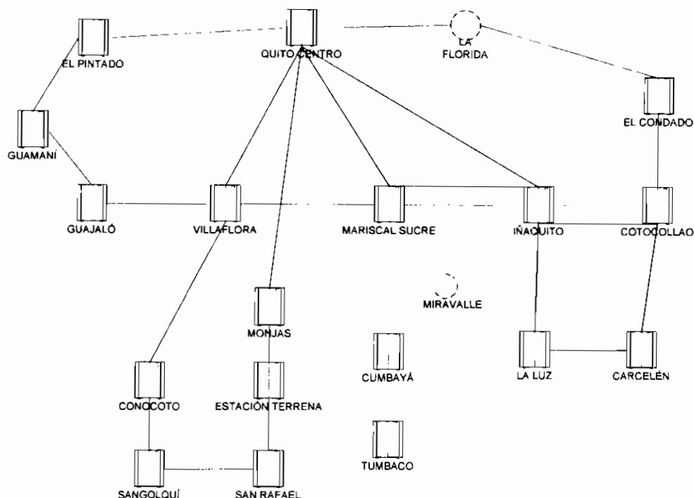
Figura 1.15 Red de Transporte – Interconexión entre anillos.
