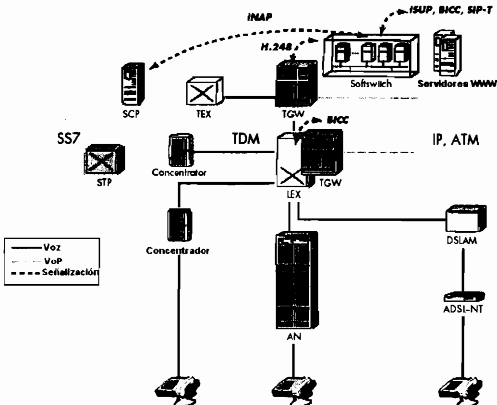
Figura 3.14 Encaminamiento de Voz sobre Paquetes VoP [37]
