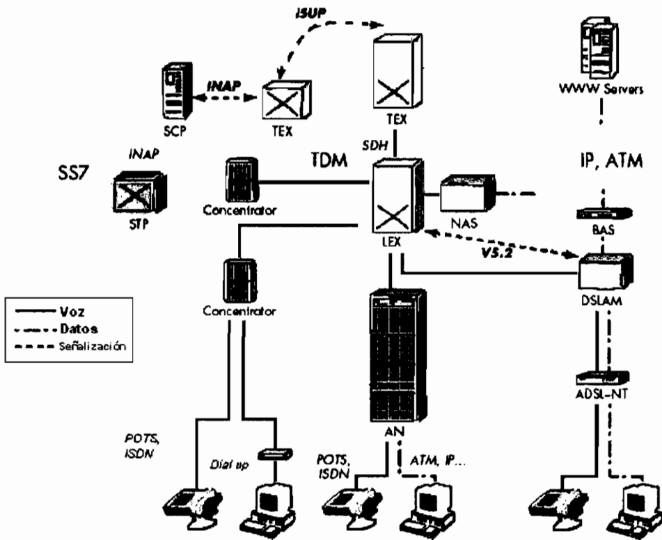
Figura 3.1 Esquema de la red actual PSTN de Andinatel en Quito [37].
