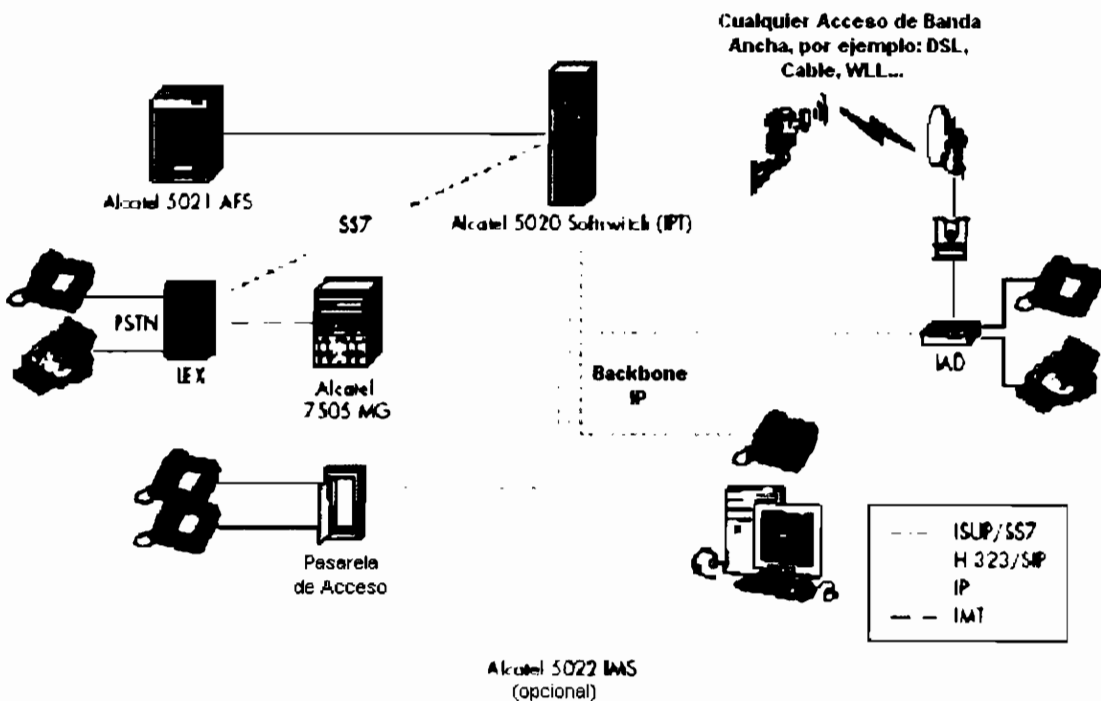
Figura 3.11 Configuración de Red con Aplicación IPT [10].
