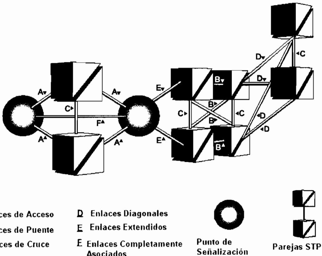
Figura 1.13 Arquitectura SS7 [33]
