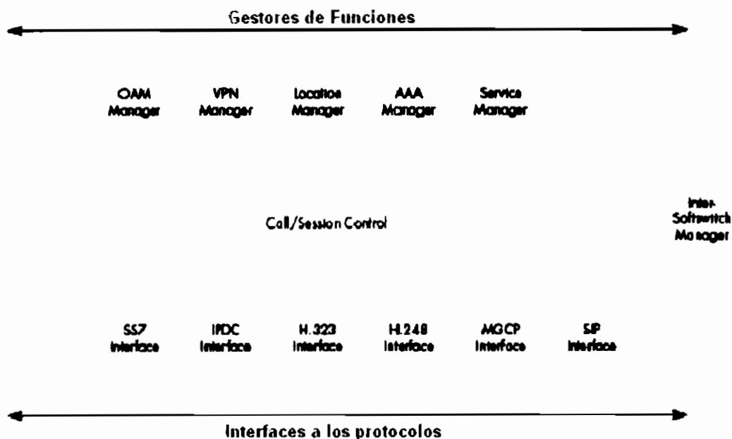
Figura 3.8 Arquitectura del Software del Softswitch 5020 [39].
