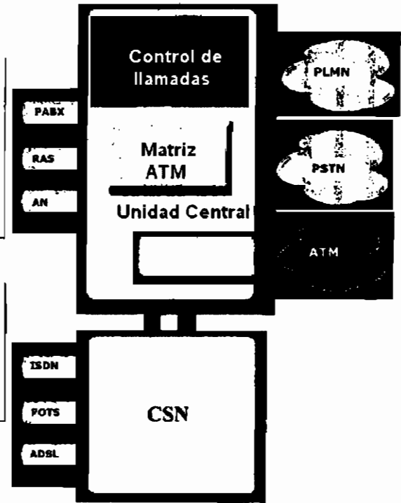
Figura 3.2 Características de una plataforma Next Generation Switch (NGS) de Alcatel [40].
