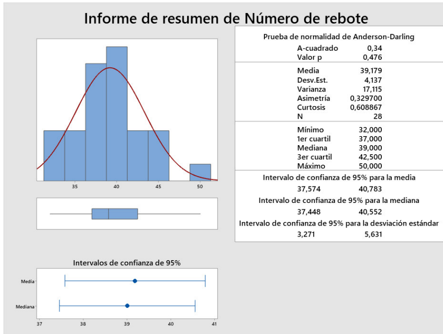
Figura 54. Análisis de datos – ensayo de esclerómetro
