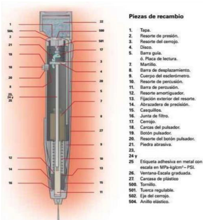
Figura 10. Corte transversal del esclerómetro
