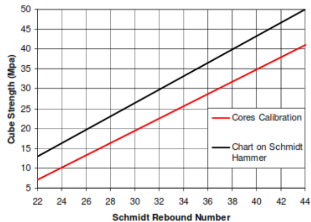
Figura 20. Comparación de curvas obtenidas de edificios existentes y compañías manufactureras
