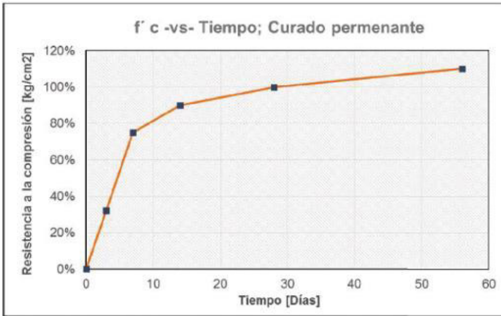
Figura 5. Crecimiento de la resistencia del hormigón
