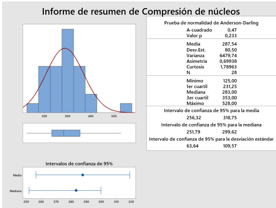
Figura 56. Análisis de datos – ensayo de compresión de núcleos Fuente: elaboración propia
