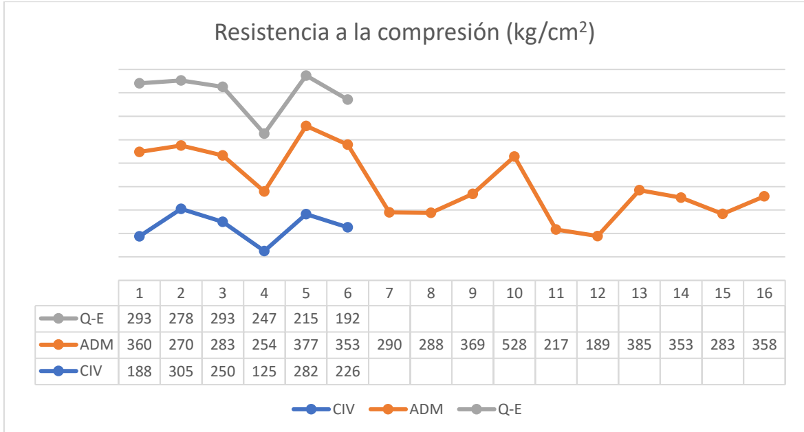
Figura 62. Resistencia a la compresión por edificio estudiado Fuente: elaboración propia
