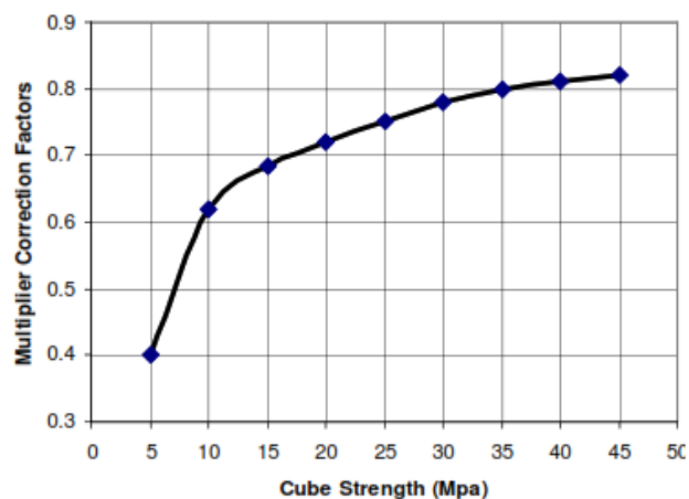
Figura 21. Factores de corrección de resistencia para la prueba de rebote
