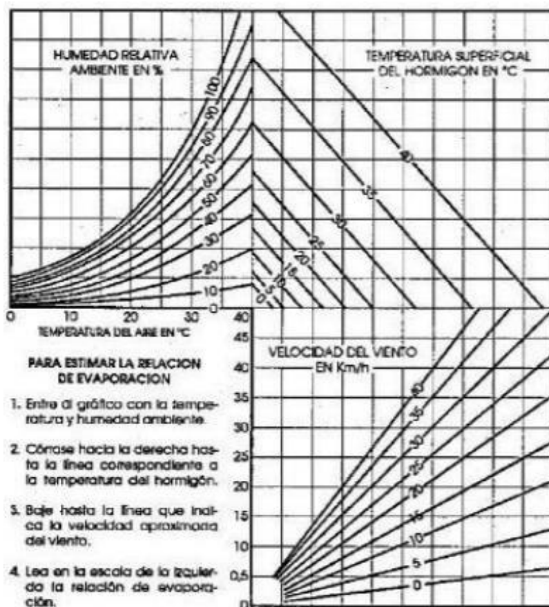
Figura 8. Cantidad de agua evaporada del hormigón en función de la humedad relativa ambiental, temperatura superficial del hormigón y velocidad del viento Fuente: (American Concrete Institute, 1991)
