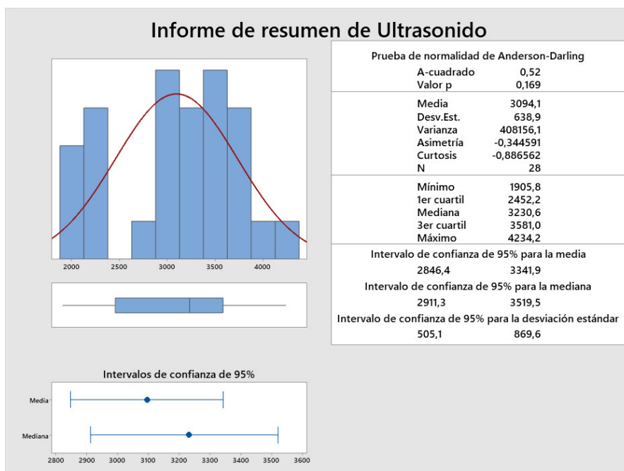
Figura 55. Análisis de datos – ensayo de ultrasonido
