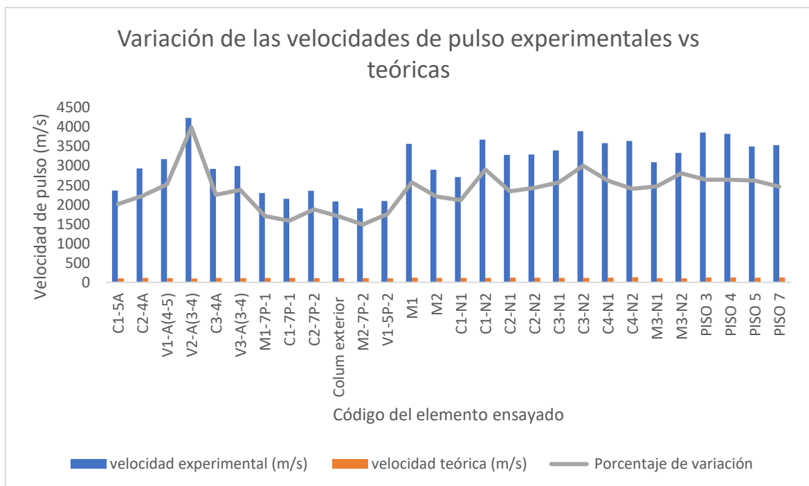
Figura 61. Variación de las velocidades de pulso experimentales vs teóricas Fuente: elaboración propia
