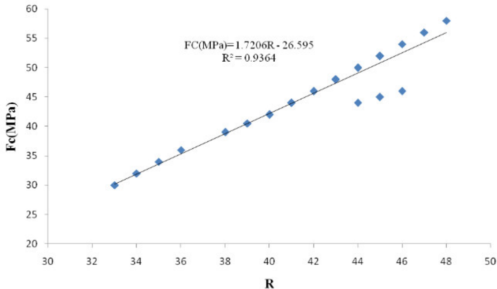
Figura 25. Curva de correlación número de rebote/resistencia a la compresión Fuente: (Shariati et al., 2011)
