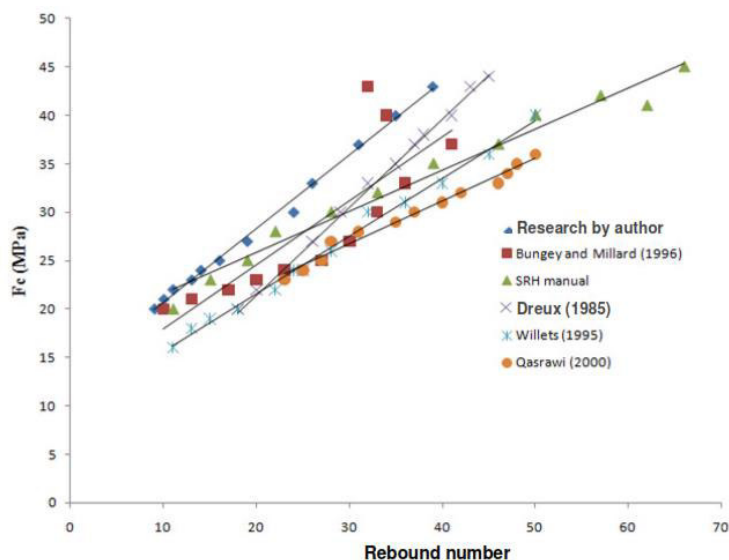
Figura 27. Comparación de resultados de la prueba del Martillo de Rebote Schmidt con otros autores
