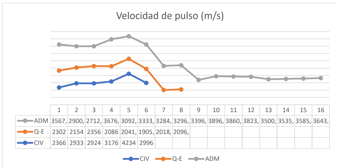
Figura 60. Velocidad de pulso por edificio estudiado Fuente: elaboración propia
