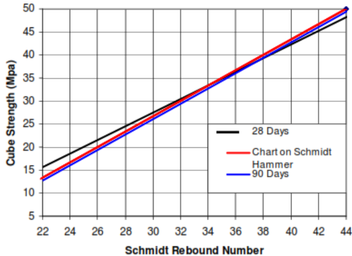
Figura 18. Relación entre el número de rebote y la resistencia cúbica de varios especímenes de diferentes edades Fuente: (Aydin & Saribiyik, 2010)
