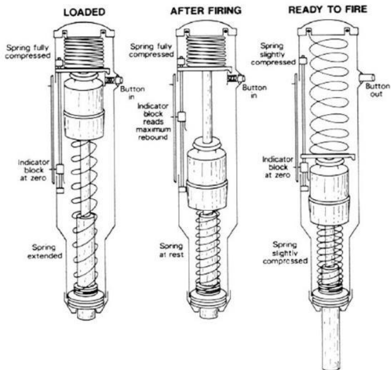
Figura 22. Sistema operativo del martillo de rebote utilizado Fuente: (Shariati et al., 2011)
