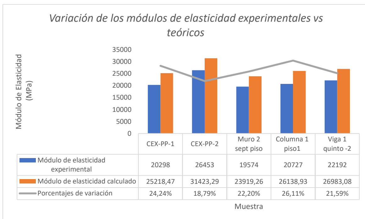
Figura 70. Variación de los módulos de elasticidad experimentales vs teóricos Fuente: elaboración propia
