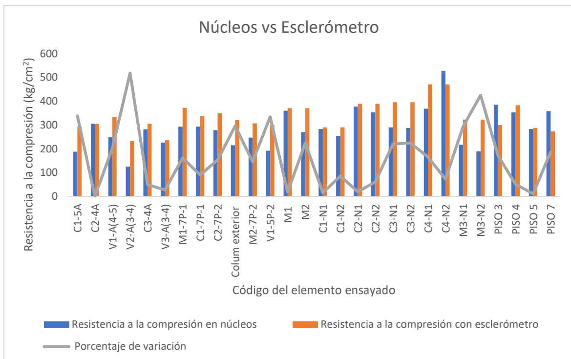
Figura 63. Variación de la resistencia a la compresión en núcleos vs esclerómetro Fuente: elaboración propia
