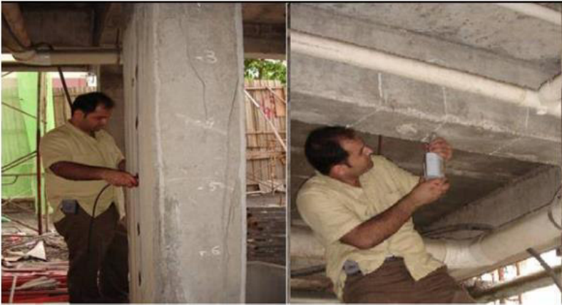
Figura 24. Ensayo de ultrasonido (izq.) y Ensayo de esclerómetro (der.) in situ Fuente: (Shariati et al., 2011)
