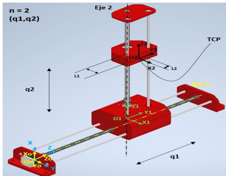
Figura 3.7. Definición de Sistemas coordenados con Denavit-Hartenberg.
