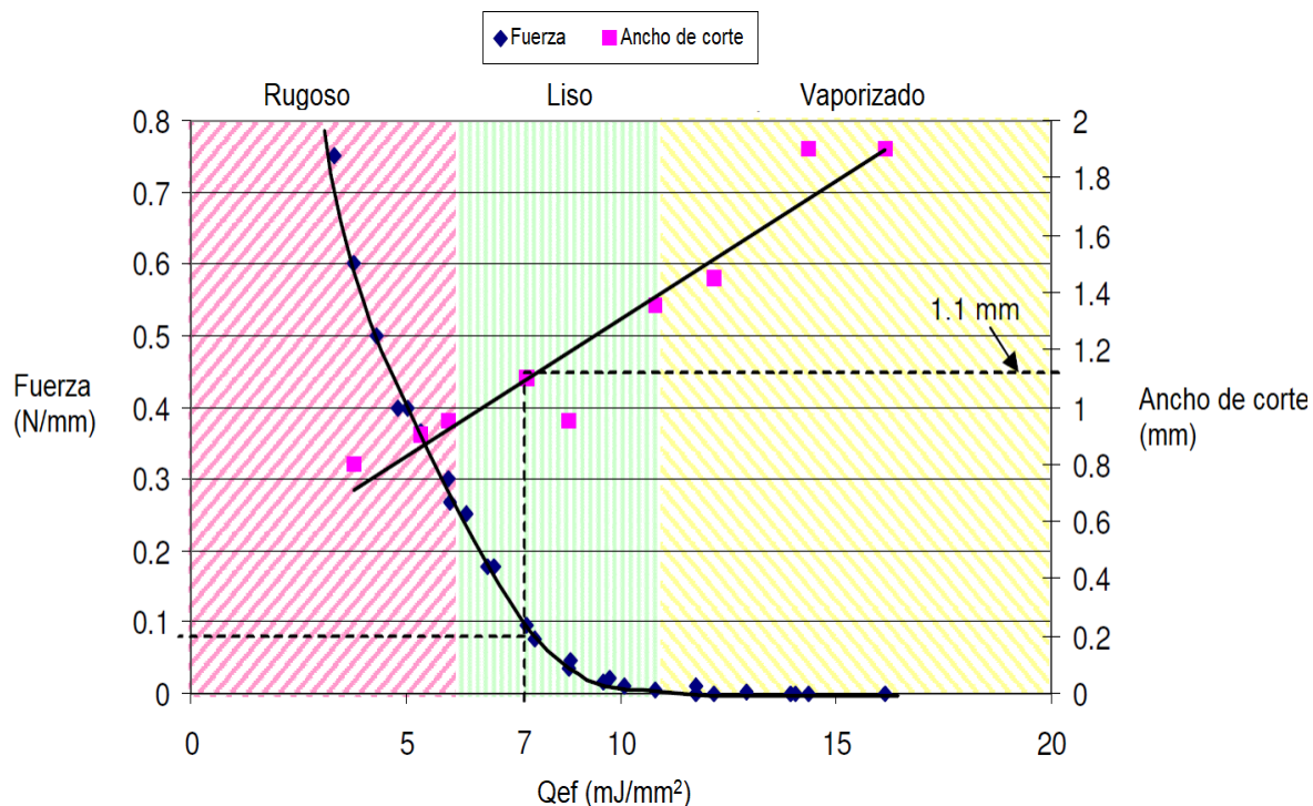
Figura 1.20. Fuerza y ancho de corte vs. entrada de calor efectiva para EPS de grado VH para un alambre de nicromo de 0,64 mm de diámetro.
