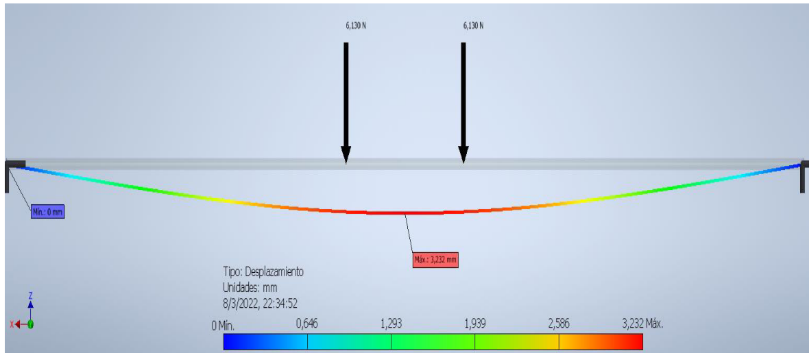
Figura 3.14. Deflexión máxima del eje guía \varnothing 8 mm L800 mm. (Fuente: Propia)
