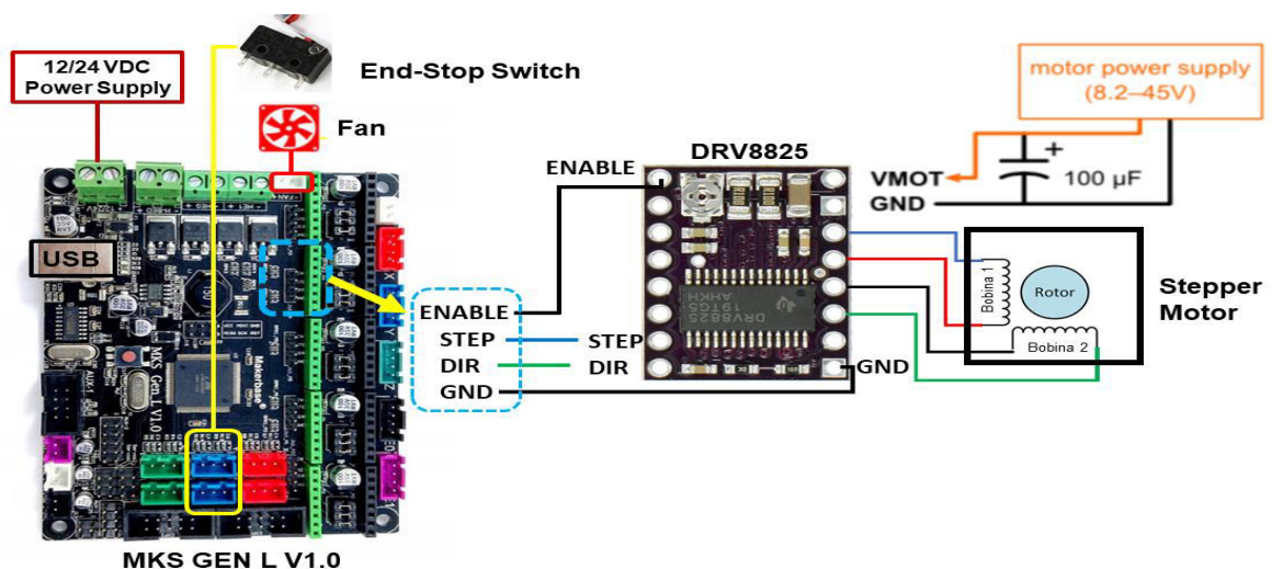
Figura 3.23. Diagrama de conexión electrónica. (Fuente: Propia)
