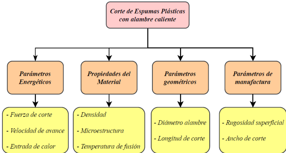
Figura 1.13. Parámetros relevantes en el corte de espumas plásticas con alambre caliente. (Fuente: Propia)
