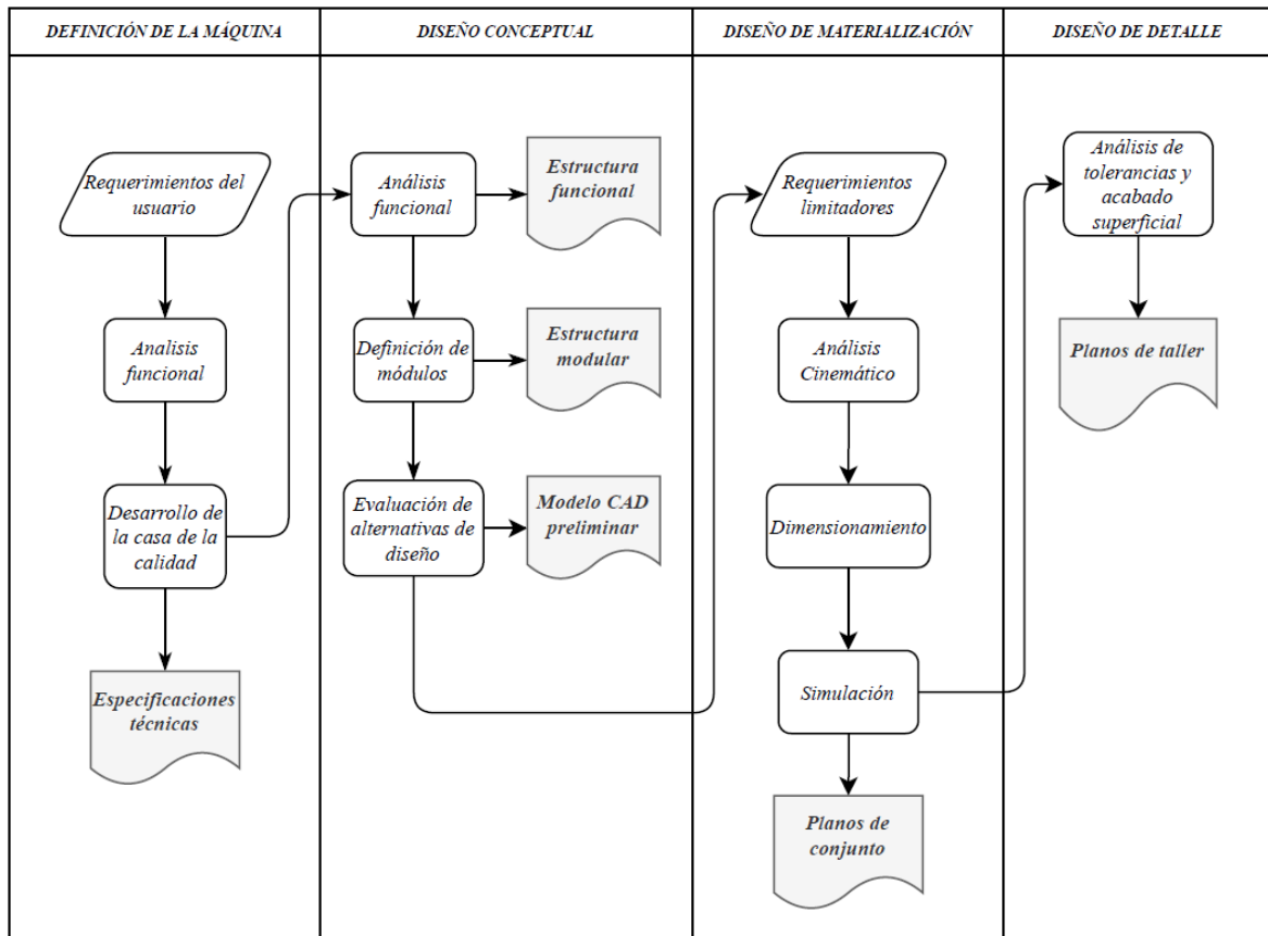
Figura 2.1. Diagrama de Flujo de la metodología para el diseño de la cortadora CNC de poliestireno.
