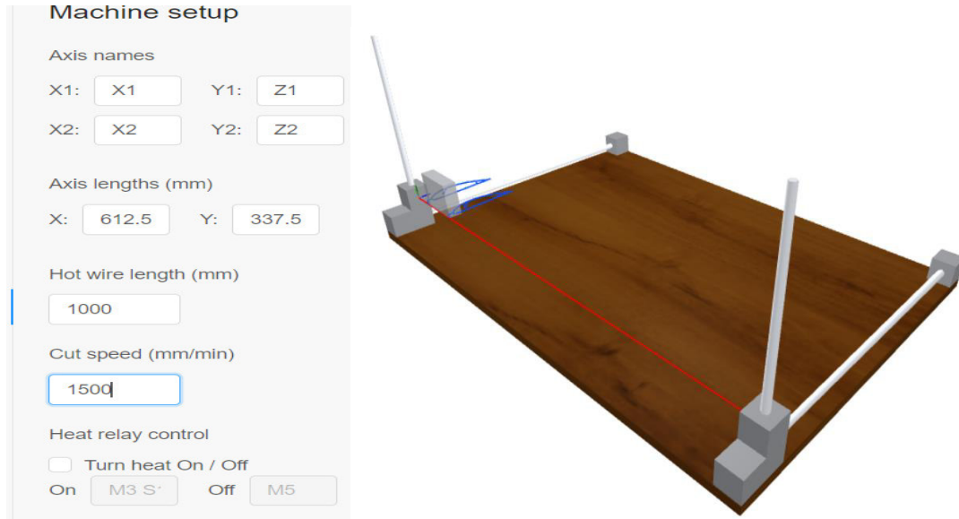
Figura 3.31. Configuración de los parámetros de la máquina. (Fuente: Propia)
