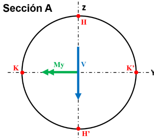
Figura 3.12. Análisis en el punto crítico en la sección crítica A.
