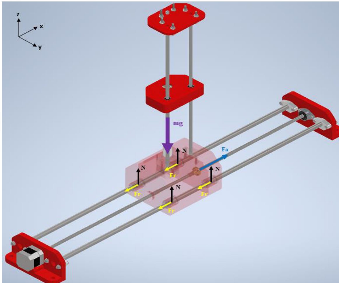
Figura 3.17. DCL para el cálculo de la fuerza axial en el tornillo de avance eje X.
