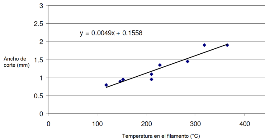
Figura 1.19. Ancho de corte vs temperatura del alambre para el corte de espuma EPS con un alambre de nicromo de 0,64 mm de diámetro.
