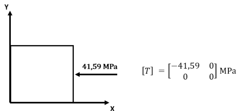
Figura 3.13. Estado de esfuerzo plano XY en el punto H.
