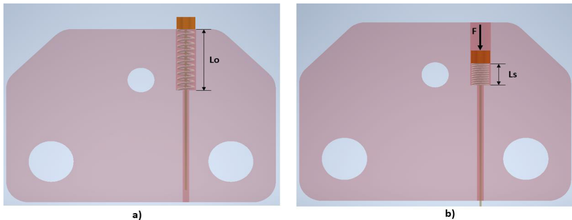
Figura 3.21. Vista superior del mecanismo de tracción y sujeción del alambre de corte en el carro vertical derecho. (Fuente: Propia)
