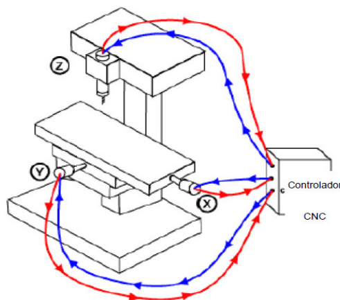
Figura 1.4. Control en lazo cerrado.
