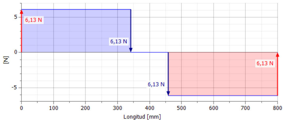
Figura 3.10. Diagrama cortante Plano XZ.
