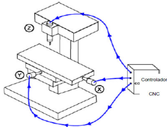
Figura 1.3. Control en lazo abierto.
