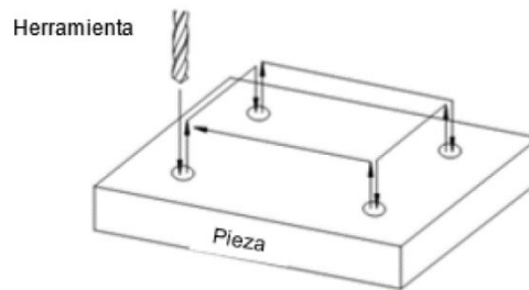
Figura 1.1. Sistema punto a punto. (Fuente: [9])
