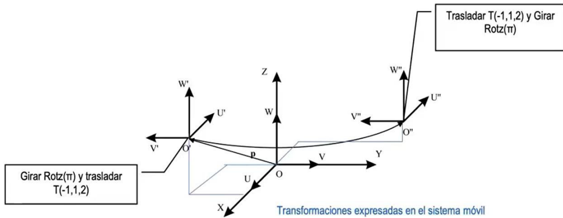
Figura 1.24. Transformación definida sobre un sistema móvil (OUVW). (Fuente: [21])
