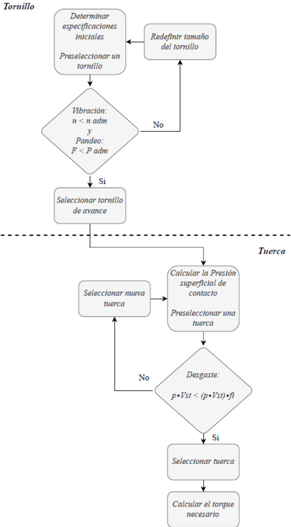
Figura 3.16. Ruta de cálculo para el dimensionamiento del tornillo de avance y tuerca. (Fuente: Propia)
