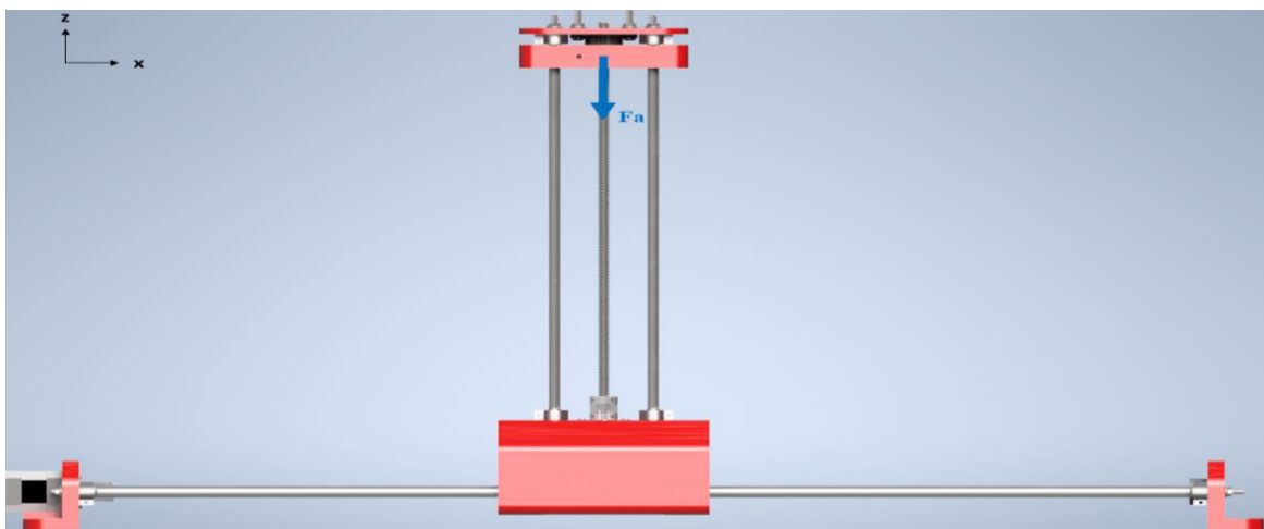
Figura 3.18. Diagrama de cuerpo libre del mecanismo vertical (Eje Z) de la máquina.
