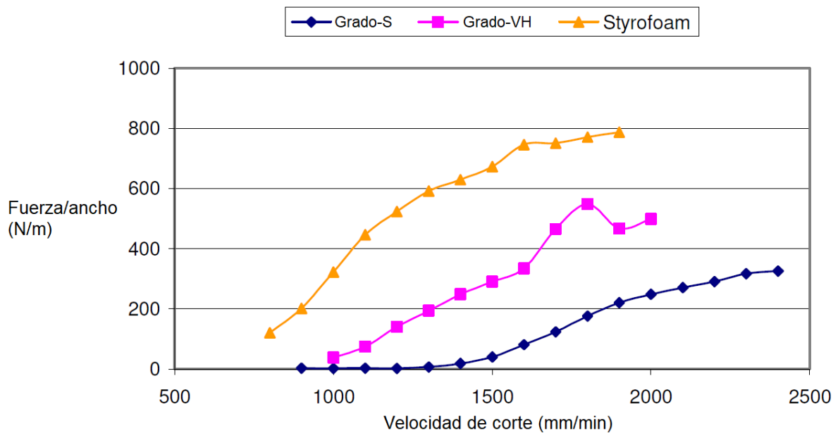
Figura 1.16. Fuerza de corte vs. velocidad de corte para diferentes tipos de espumas con 6A. (Fuente:[1])
