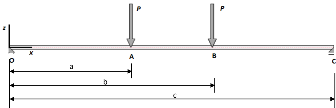
Figura 3.9. Diagrama de cuerpo libre del eje guía.
