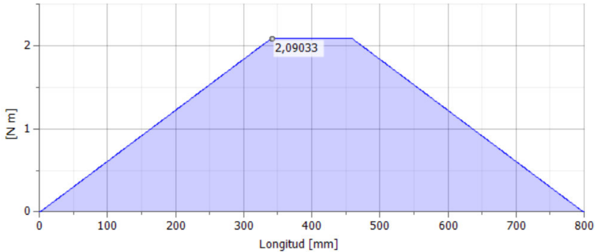
Figura 3.11. Diagrama momento flector plano XZ.
