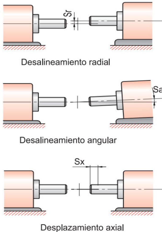
Figura 3.19. Tipos de desalineación.
