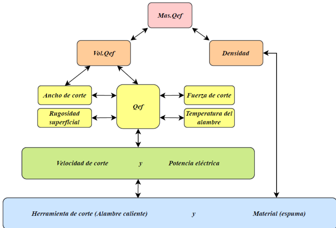
Figura 1.21. Resumen de las relaciones entre los parámetros de corte de la espuma. (Fuente: Propia)
