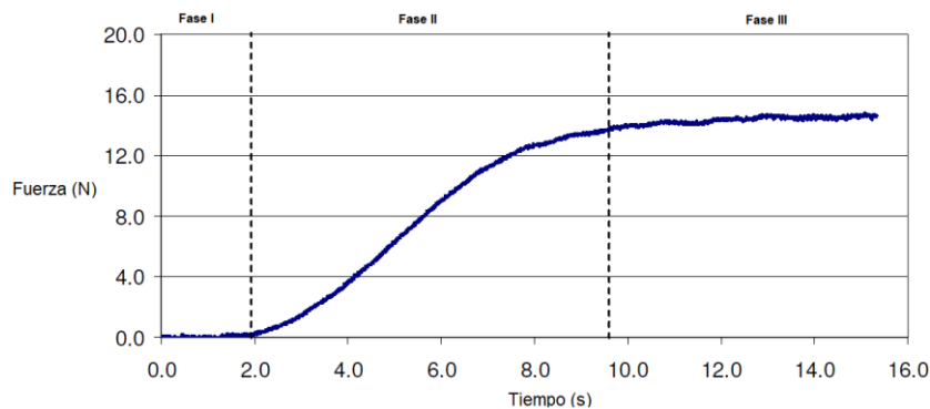
Figura 1.14. Curva característica de la fuerza de corte para una muestra de XPS (5A - 0.02 m/s). (Fuente:[1])
