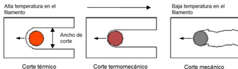
Figura 1.11. Mecanismo de corte y "kerf" asociado. (Fuente: [1])
