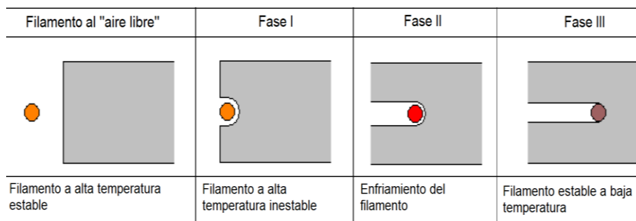
Figura 1.12. Fases de corte.
