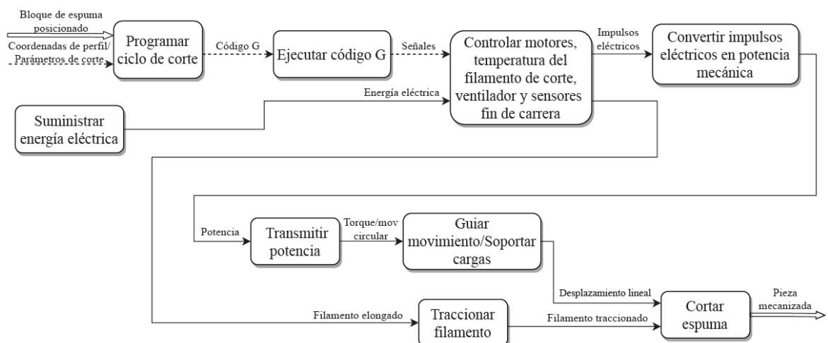
Figura 3.4. Nivel 2 del análisis funcional – estructura funcional.
