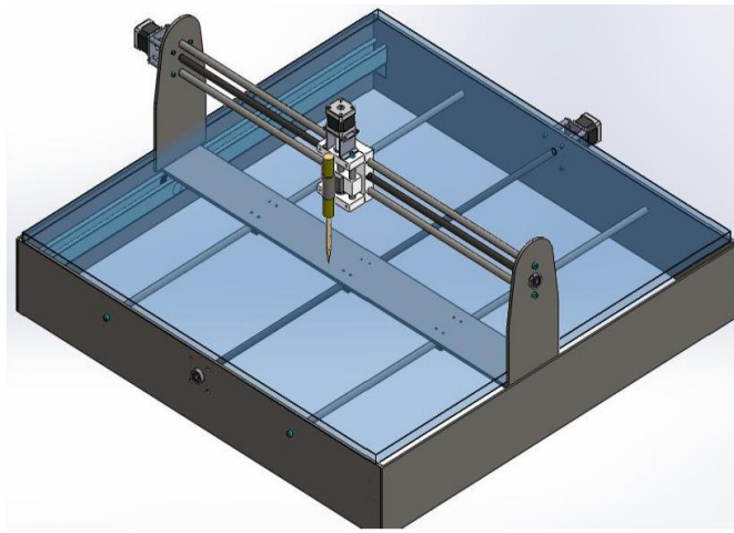
Figura 1.9. Máquina CNC de tres ejes.
