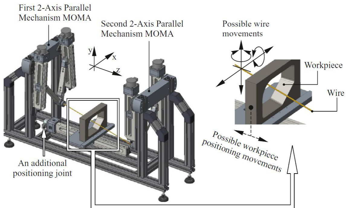
Figura 1.5. Modelo CAD de la máquina reconfigurable multi-eje en un proceso de corte por alambre caliente.
