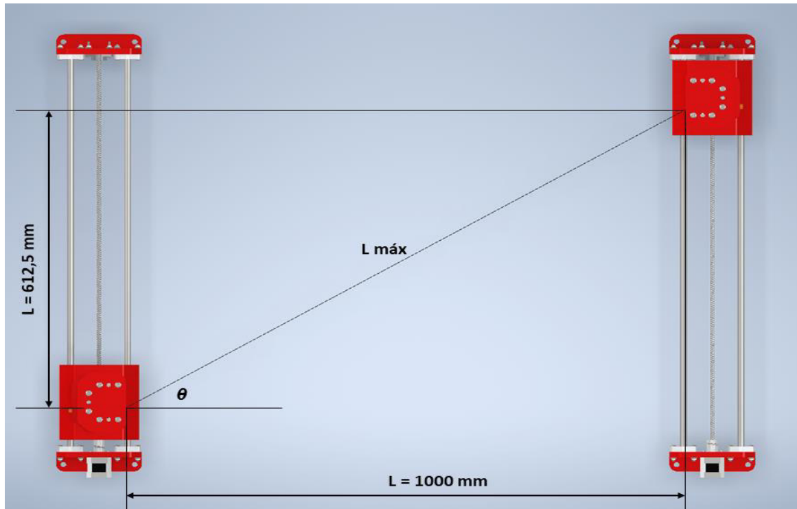
Figura 3.22. Vista superior de la máquina con un ángulo \theta máximo.
