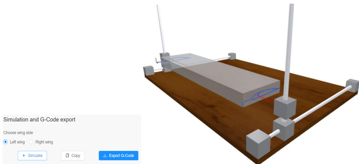
Figura 3.34. Simulación de corte.
