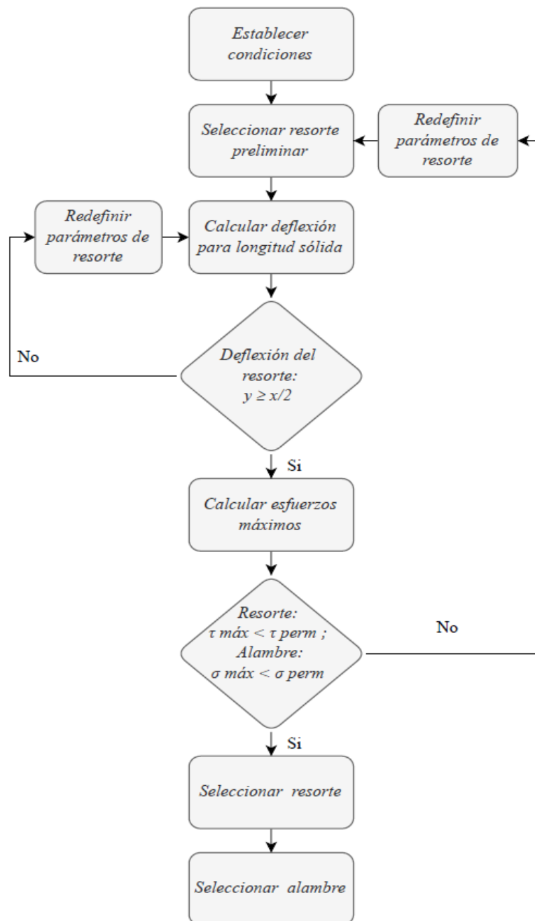
Figura 3.20. Ruta de cálculo para el dimensionamiento del resorte y alambre de corte.
