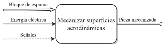
Figura 3.2. Nivel 0 del análisis funcional.
