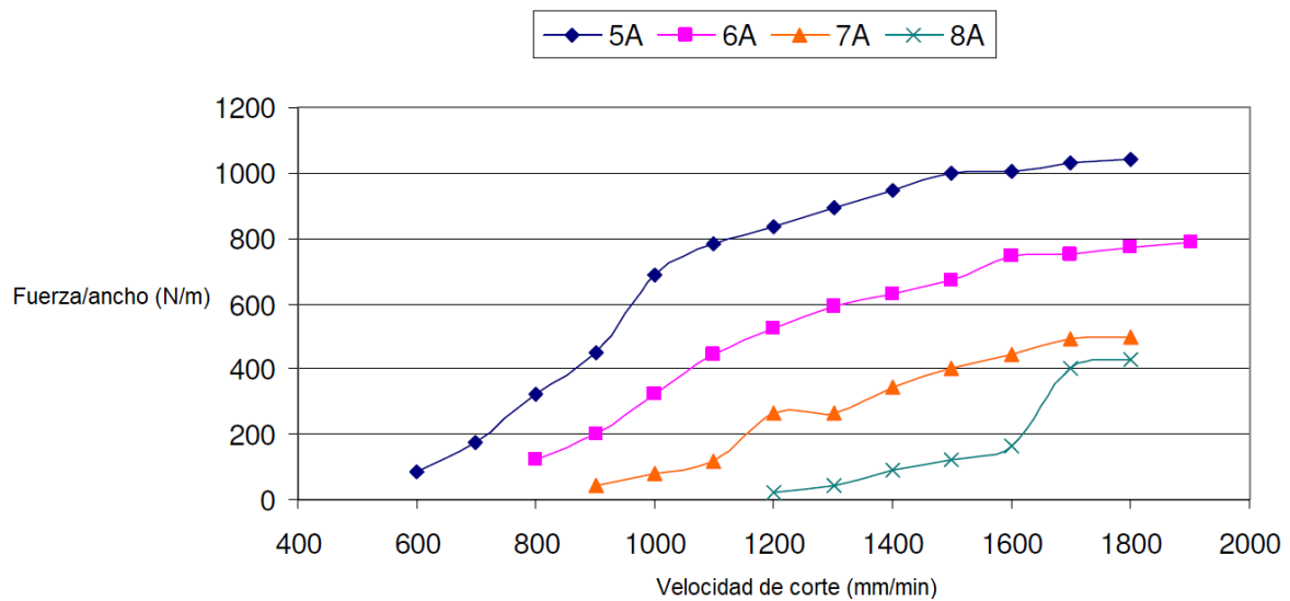
Figura 1.15. Fase III fuerza de corte vs. velocidad de corte con varias corrientes en una muestra de XPS. (Fuente:[1])
