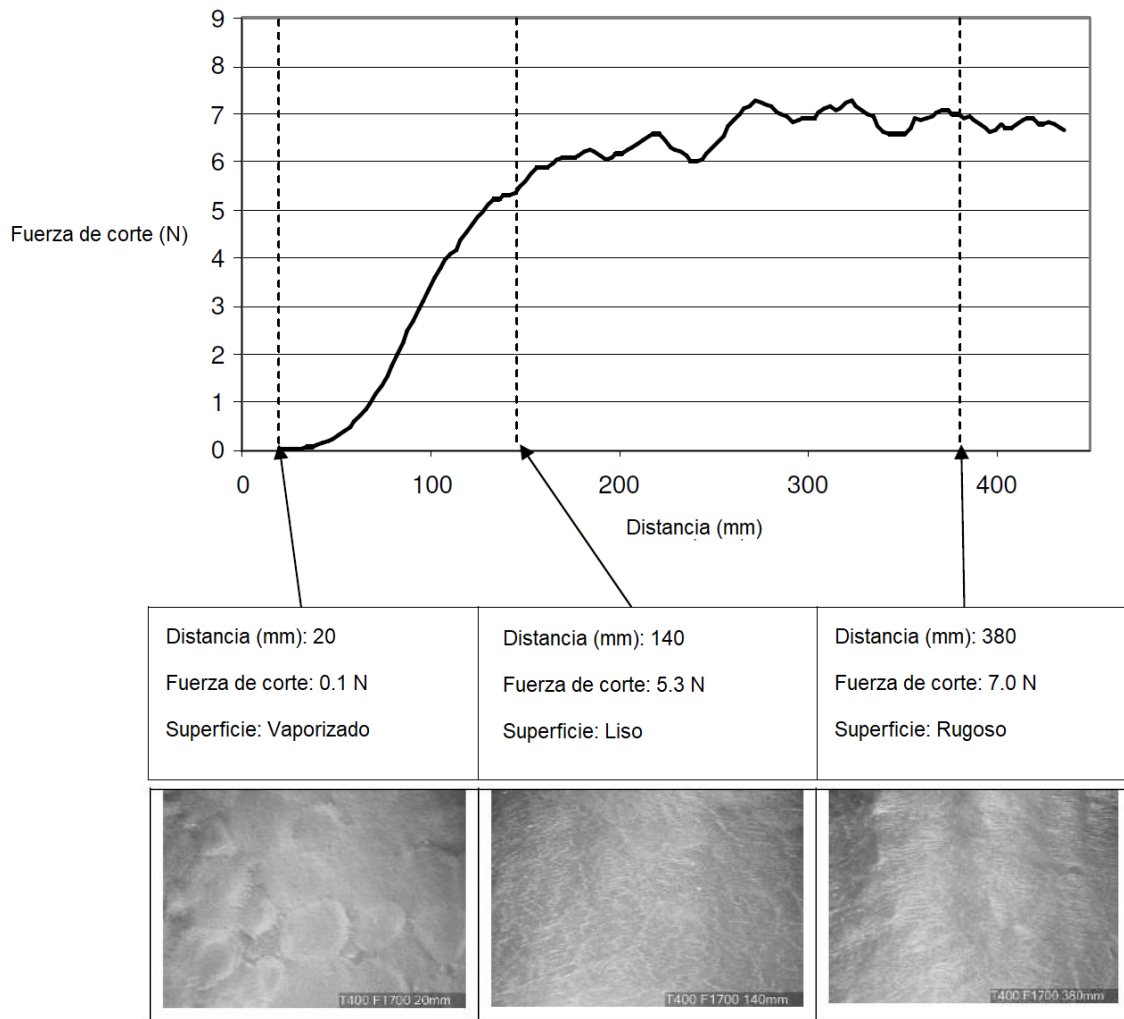
Figura 1.17. Relación fuerza de corte / acabado superficial para EPS de grado S (5A - 0,0283 m/s). (Fuente:[1])
