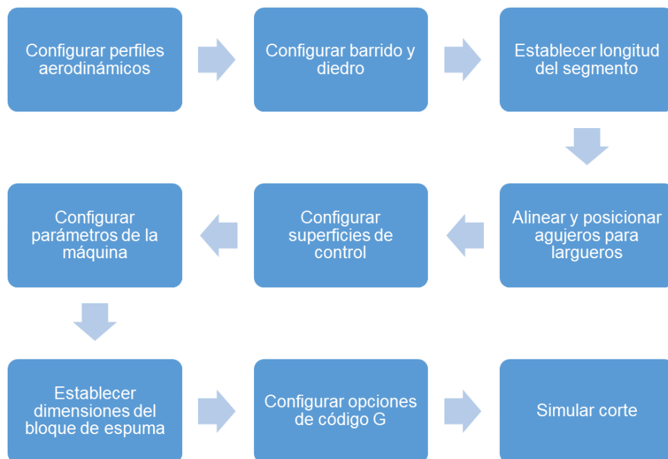
Figura 3.25. Procedimiento de simulación del corte de un ala.
