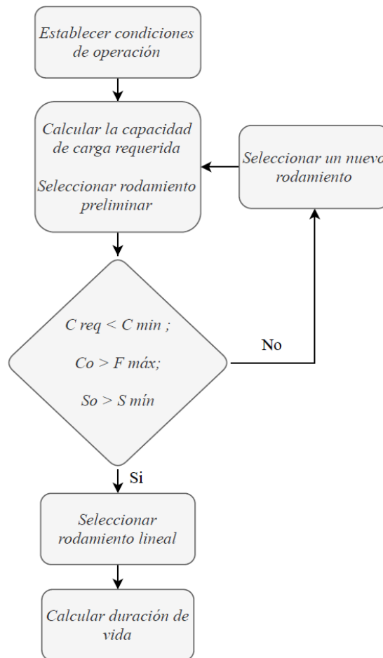
Figura 3.15. Ruta de cálculo para el dimensionamiento de los rodamientos lineales.
