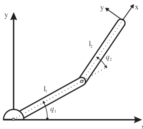
Figura 1.23. Robot con dos grados de libertad de rotación. (Fuente: [21])
