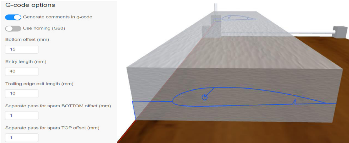
Figura 3.33. Configurar opciones de código G.
