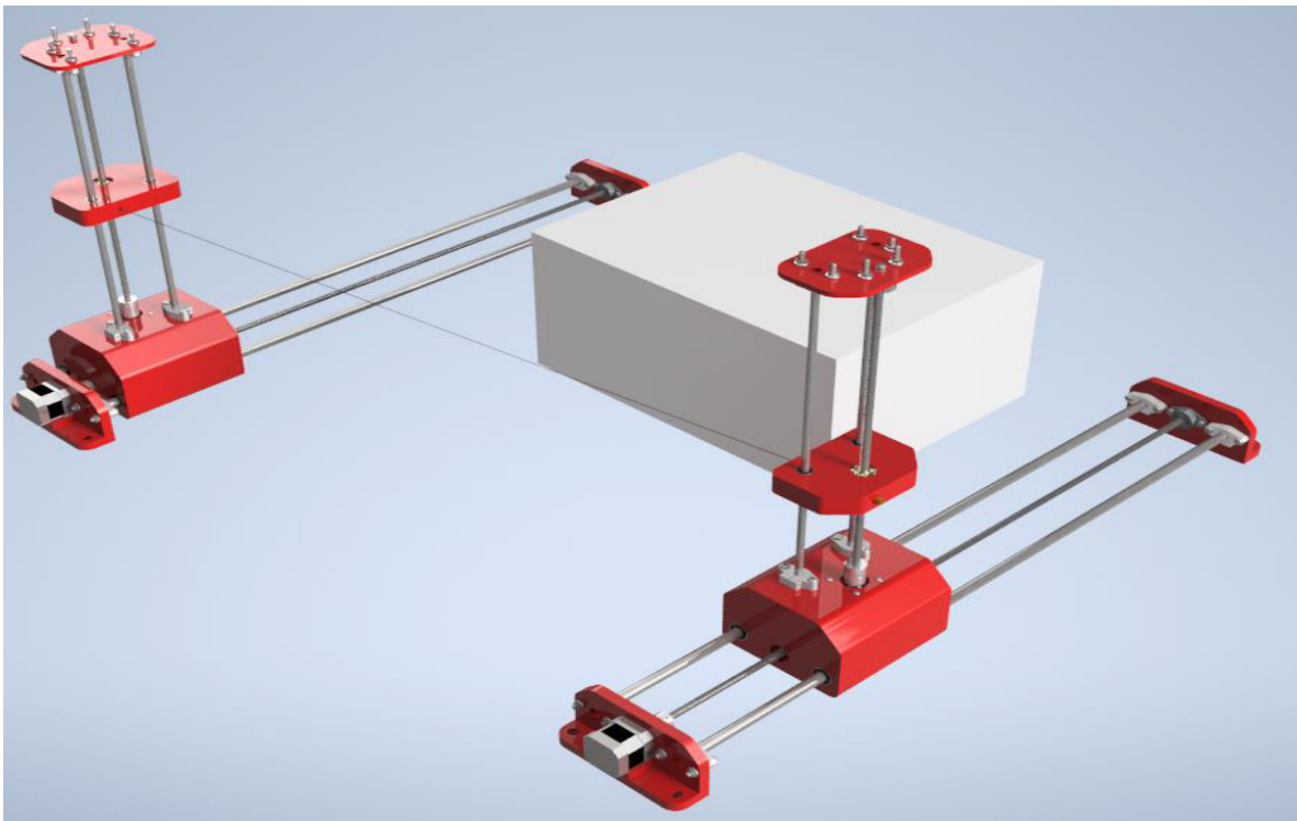
Figura 3.6. Diseño conceptual de la cortadora CNC de poliestireno.
