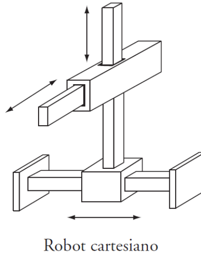
Robot cartesiano Figura 1.22. Robot cartesiano de tres grados de libertad (3GDL-PPP). (Fuente: [21])
