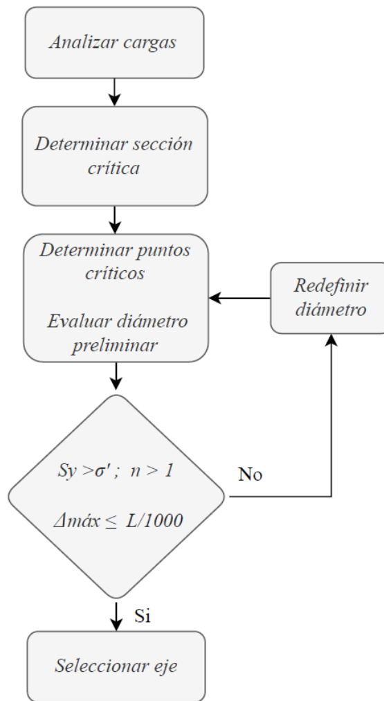
Figura 3.8. Metodología de cálculo para el eje guía.
