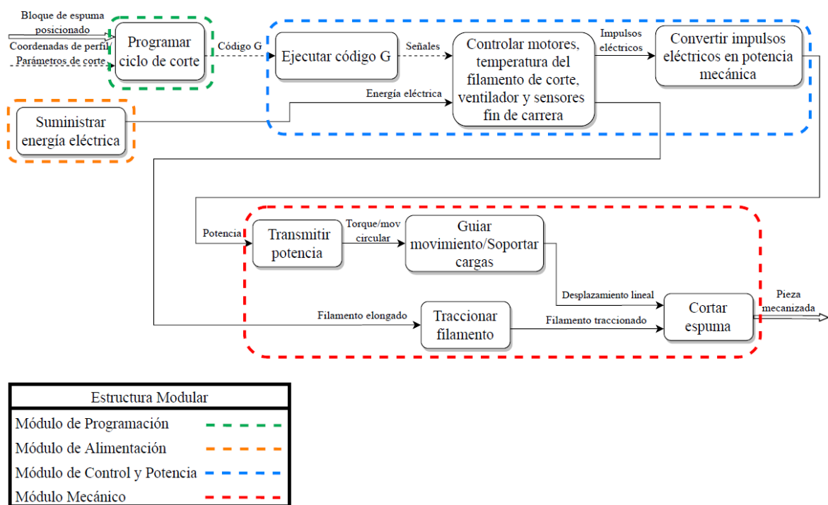
Figura 3.5. Estructura modular.
