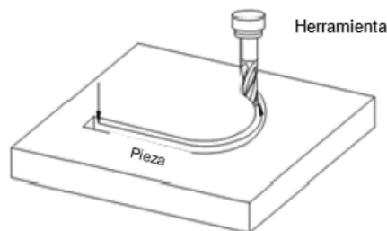
Figura 1.2. Sistema de contorno. (Fuente: [9])
