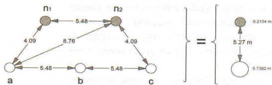
Fig. 6 Configuración línea trifásica con dos cables de guarda
