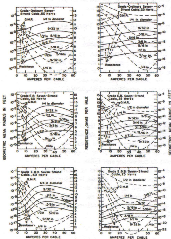
Fig. 1 Características eléctricas de los conductores de acero[4]
