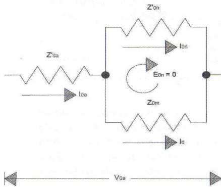
Fig. 4 Circuito equivalente para corriente de retorno de secuencia cero a través del cable de guarda y tierra
