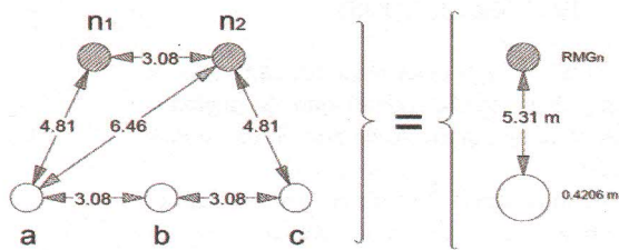
Fig. 8 Configuración línea trifásica con dos conductores de acero como cables de guarda
