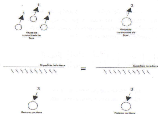
Fig. 2 Corrientes de secuencia cero
