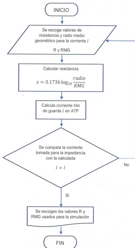
Fig. 9 Diagrama de flujo para buscar la impedancia adecuada del conductor de acero
