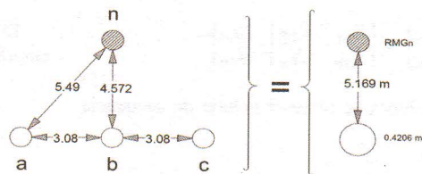
Fig. 7 Configuración línea trifásica con un conductor de acero como cable de guarda
