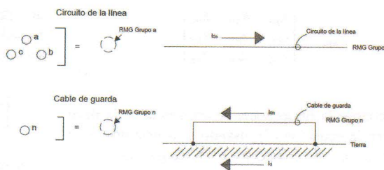
Fig. 3 Circuito para corriente de retorno de secuencia cero en el cable de guarda y tierra
