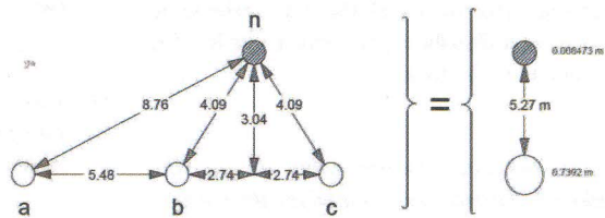
Fig. 5 Configuración línea trifásica con un cable de guarda
