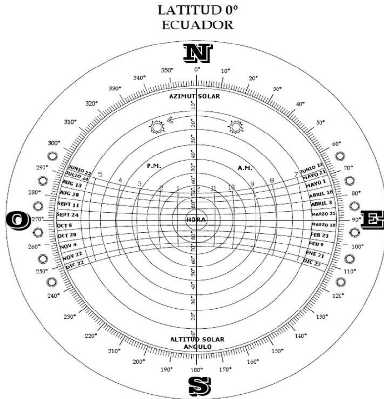
Figura 2.2. Carta solar de Ecuador [9].
