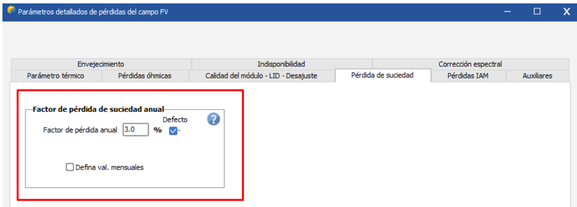
Figura 3.17. Configuración del factor de pérdidas [Elaboración Propia].
