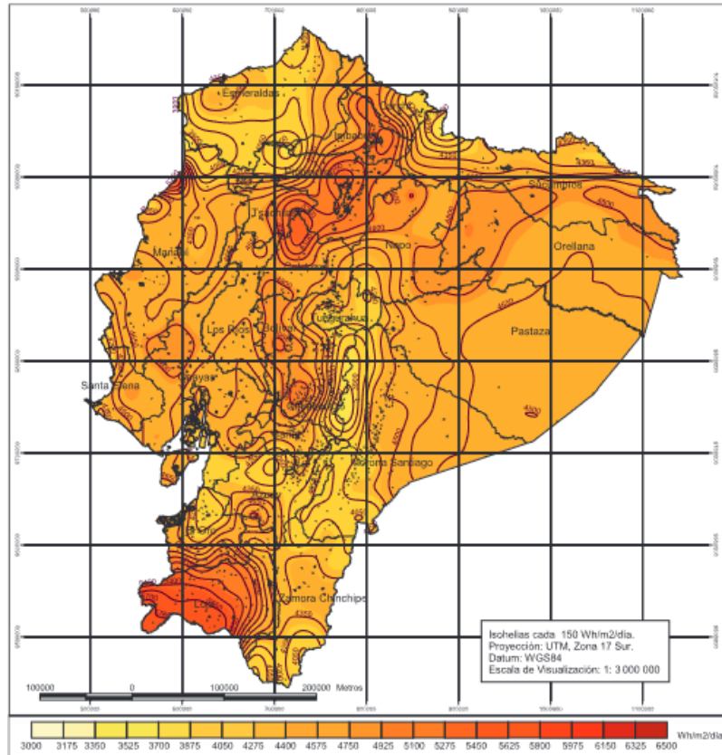
Figura 2.3. Atlas Solar del Ecuador, Radiación Global Anual [12].
