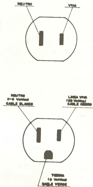
Fig. 4.- Tomacorrientes utilizados para alimentación de 110 voltios.
