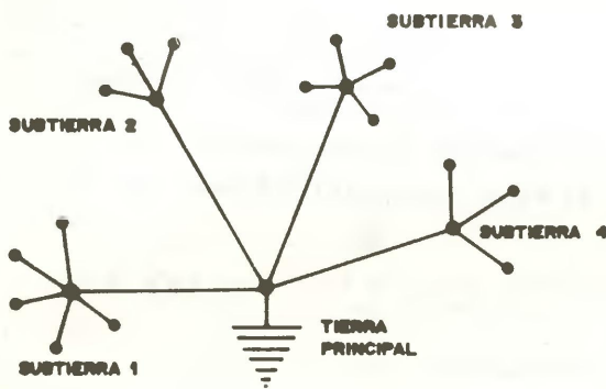
Fig. 6.- Configuración "Copo de Nieve" para las conexiones de tierra.
