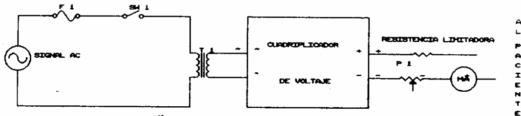
FIGURA 4.c. ESQUEMA DEL CIRCUITO DEFINITIVO.
