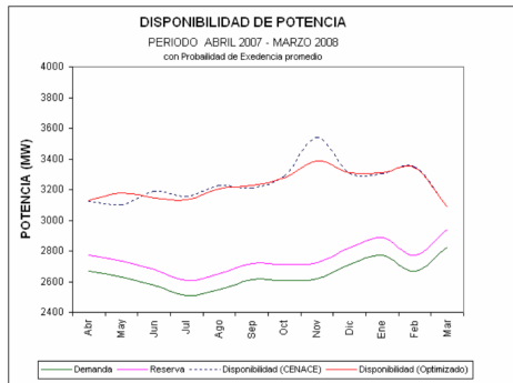
Figura 6.2.- Potencia disponible por período
