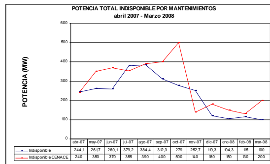
Figura 6.1.- Potencia indisponible por mantenimientos de las unidades de generación luego de la aplicación del modelo de optimización en comparación con datos CENACE
