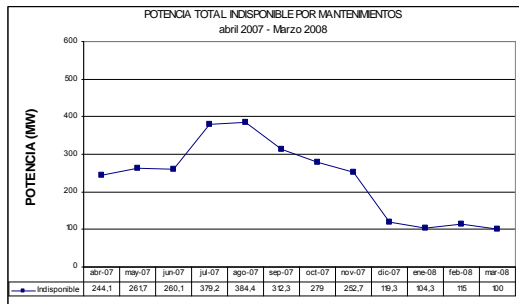
Figura 5.2.-Potencia indisponible, luego de la aplicación del modelo de optimización abril 2007 marzo 2008.
