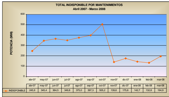
Figura 5.1.-Potencia indisponible, CENACE plan operativo abril 2007 marzo 2008
