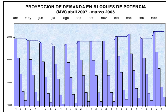
Figura 4.2. Proyección de la demanda de potencia por bloques
